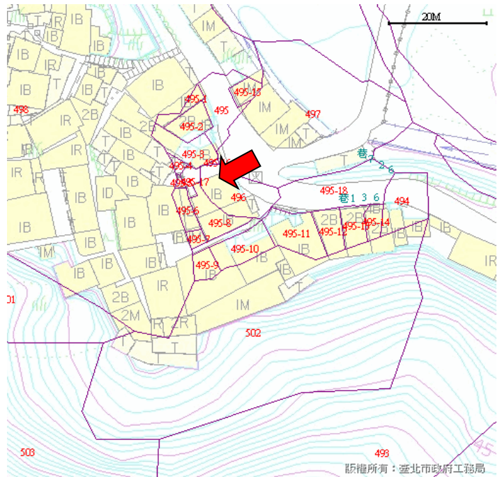
地籍圖↓
