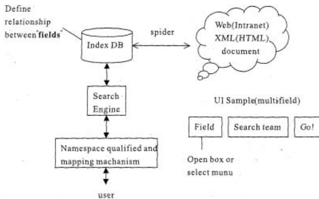
圖五:XML-based'分散式檢索引擎架構圖
