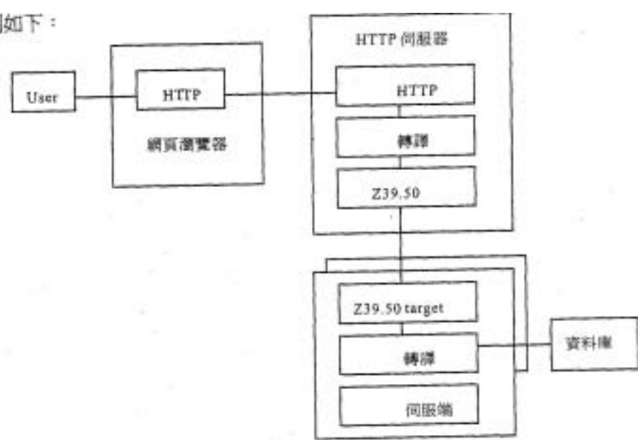
圖四：HTTP/Z39.50 gateway之系統架構
