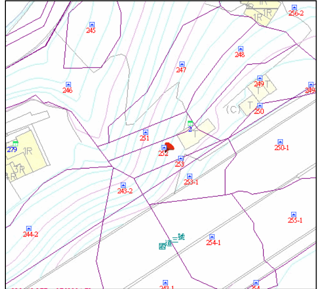
地籍圖↓
