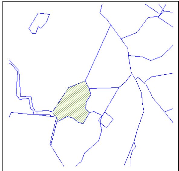
地籍圖↓
