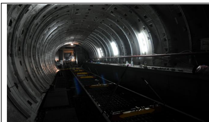
捷運環狀線大坪林站浮動式道床軌道鋪軌
