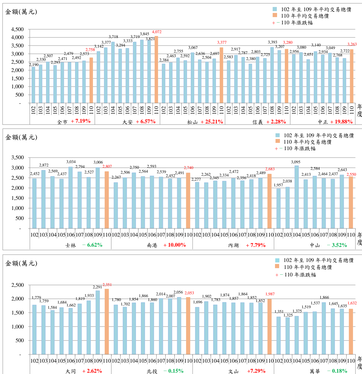
圖 8 全市及各行政區 102 至 110 年住宅平均交易總價圖
