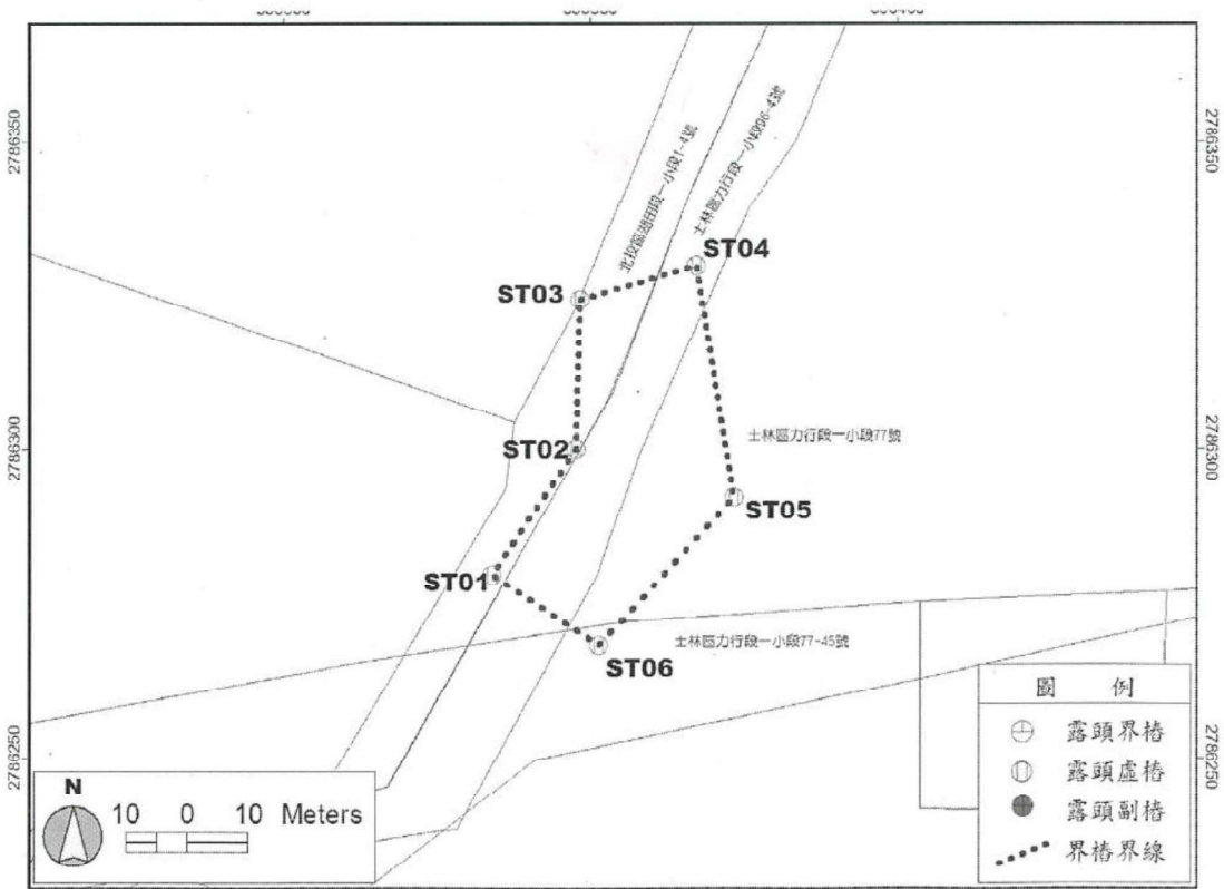
七股溫泉露頭區界樁地籍圖
