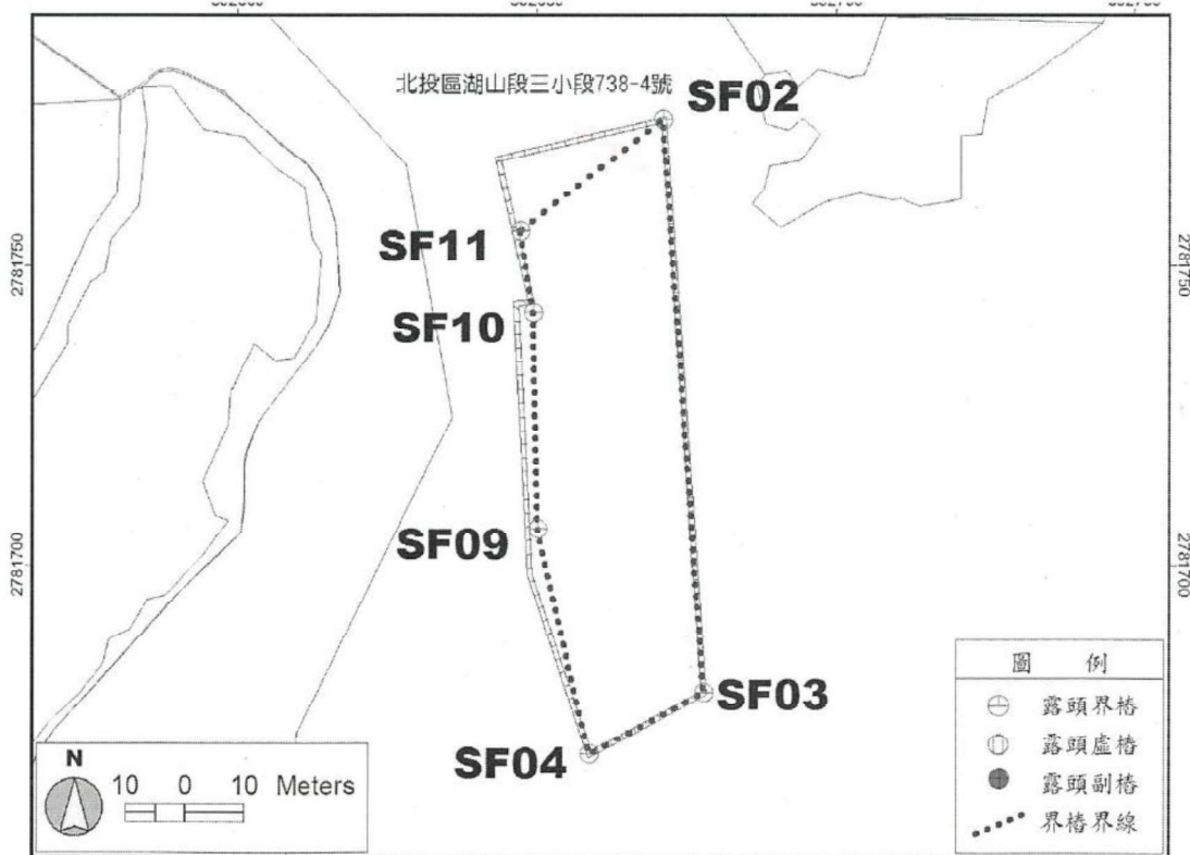
磺溪嶺 2 號溫泉露頭區界樁地籍圖
