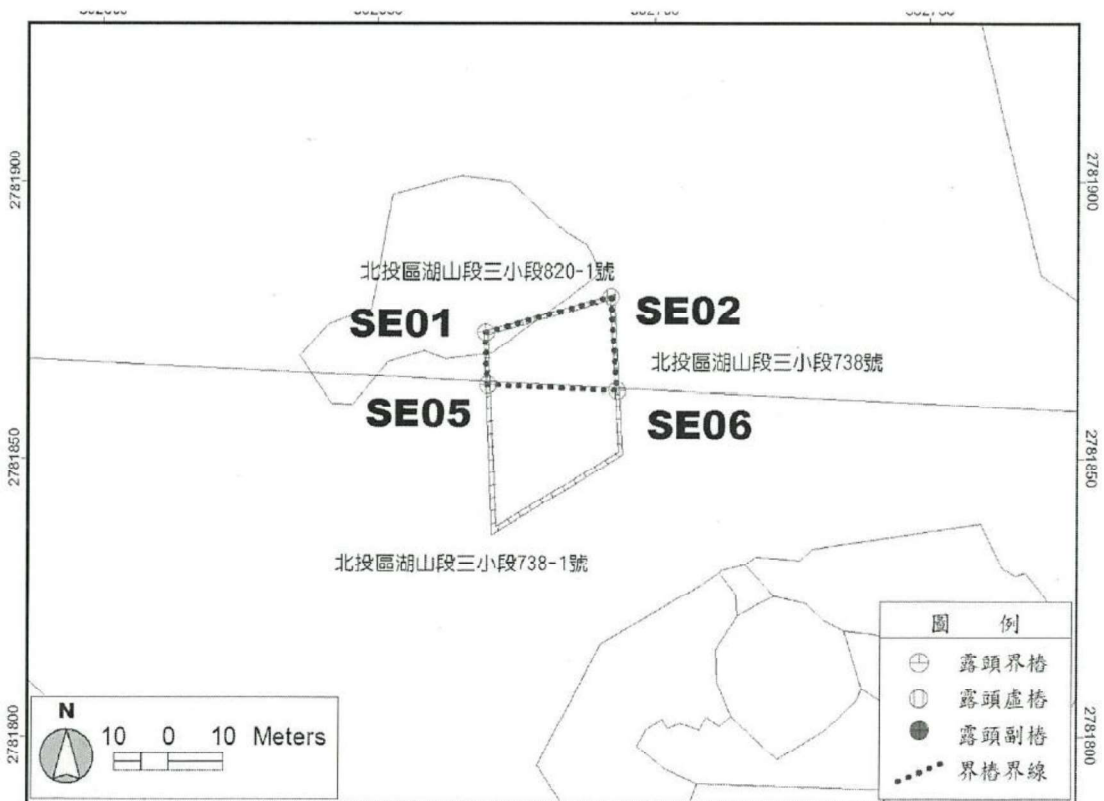
磺溪嶺 1 號溫泉露頭區界樁地籍圖
