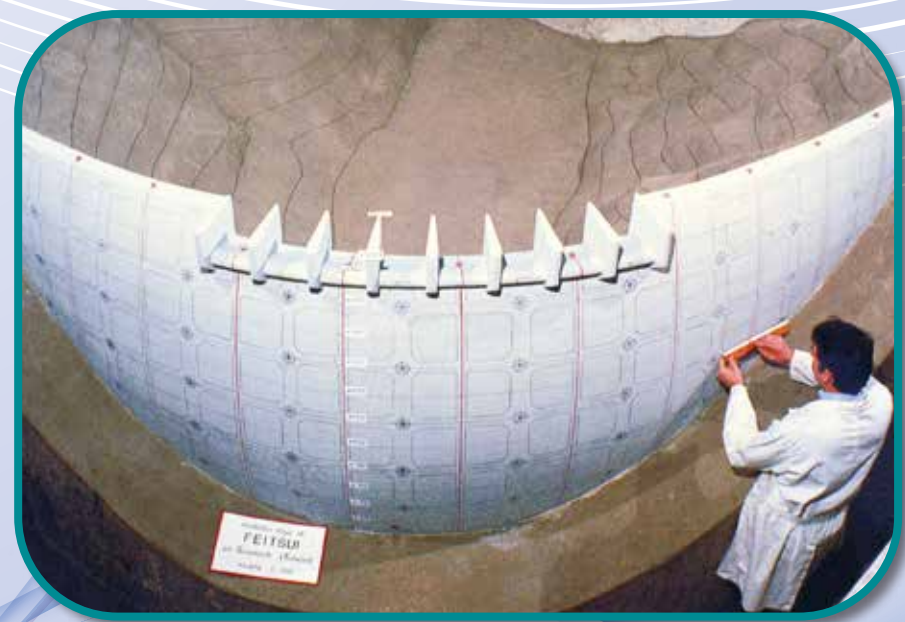
翡翠大壩結構模型（比例：1:100） 工作人員於壩體模型上游面區分油壓機施載位置
