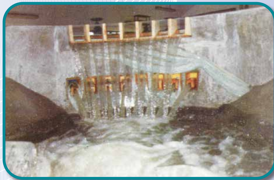
台大水工所主辦大壩溢洪道水工試驗
