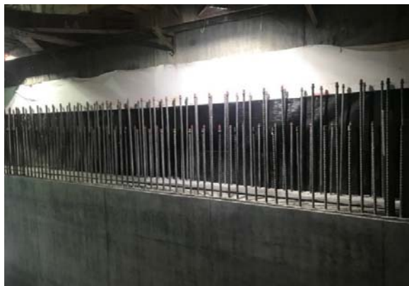
側牆鋼筋保護層及升層界面控制良好
