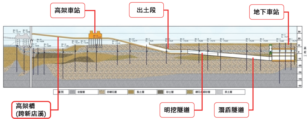
圖七、捷運環狀線CF640區段標路線縱剖面示意圖
