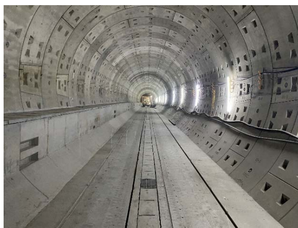
圖4 連城錦和站至中和高中站間隧道完成現況
