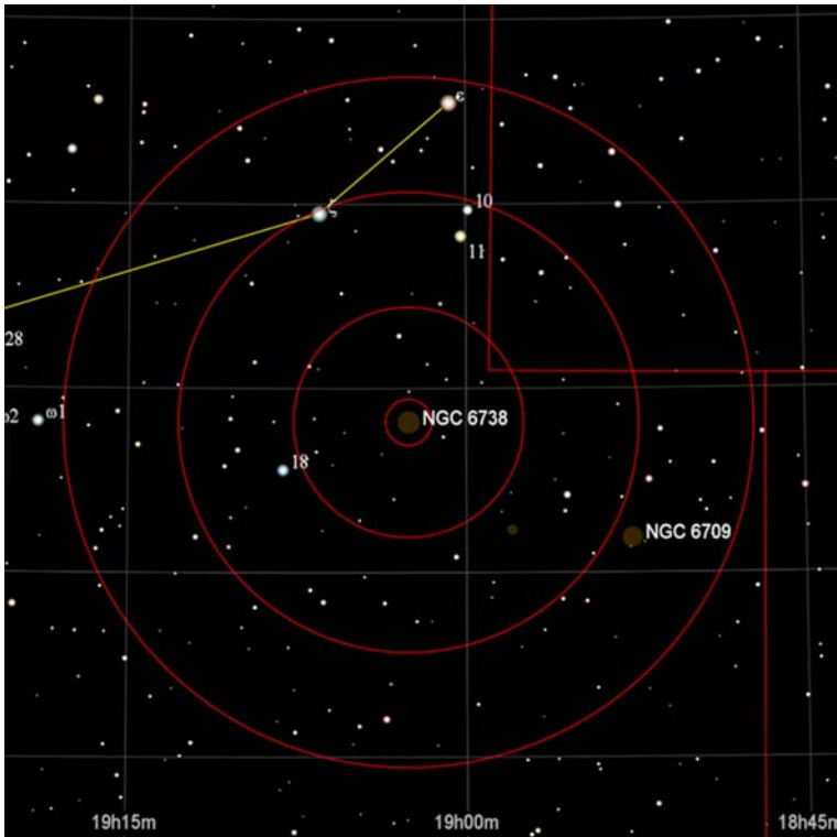
圖4. NGC 6709尋星圖。
