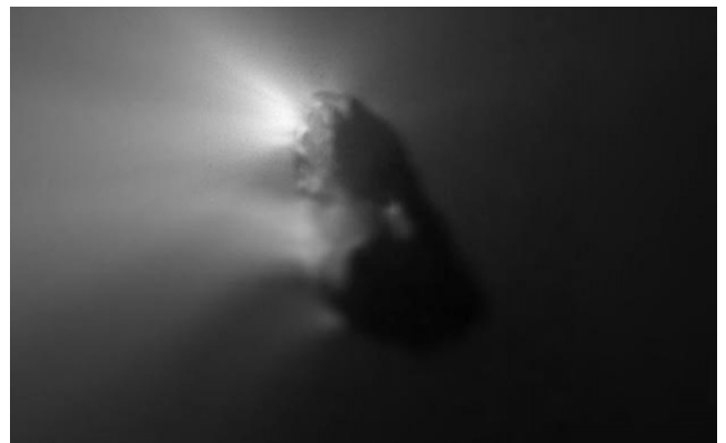
圖3. ↑↑哈雷彗星於1986年的回歸。圖片來源：NASA。↑1986年3月13日至14日間，喬托號飛到距離哈雷彗星僅596公里的地方，首次揭示了彗核近距離觀察的情況。圖片來源：ESA/Giotto/HMC
