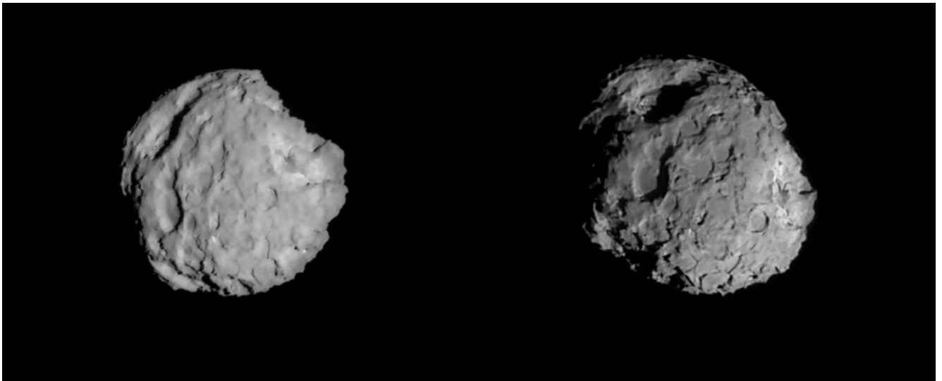
圖8. NASA 星塵號探測器上的導航相機拍攝的兩張彗星 81P/Wild 2 影像。來源影像拍攝於 2004 年 1 月 2 日 19:21:28 和 19:21:48，距離分別為 237 公里和 257 公里。圖片來源：NASA/NSSDC
