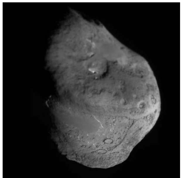
圖9. 「深度撞擊」偵測器撞擊坦普爾1號彗星表面之前的情況。由偵測器的撞擊器瞄準感測器拍攝的影像合成。撞擊地點在彗星中心和底部附近的兩個黑邊隕石坑之間。此圖像是於撞擊發生約4秒前距離彗星表面幾公尺處，所拍攝的高解析度影像。圖片來源：NASA/ JPL/ University of Maryland
