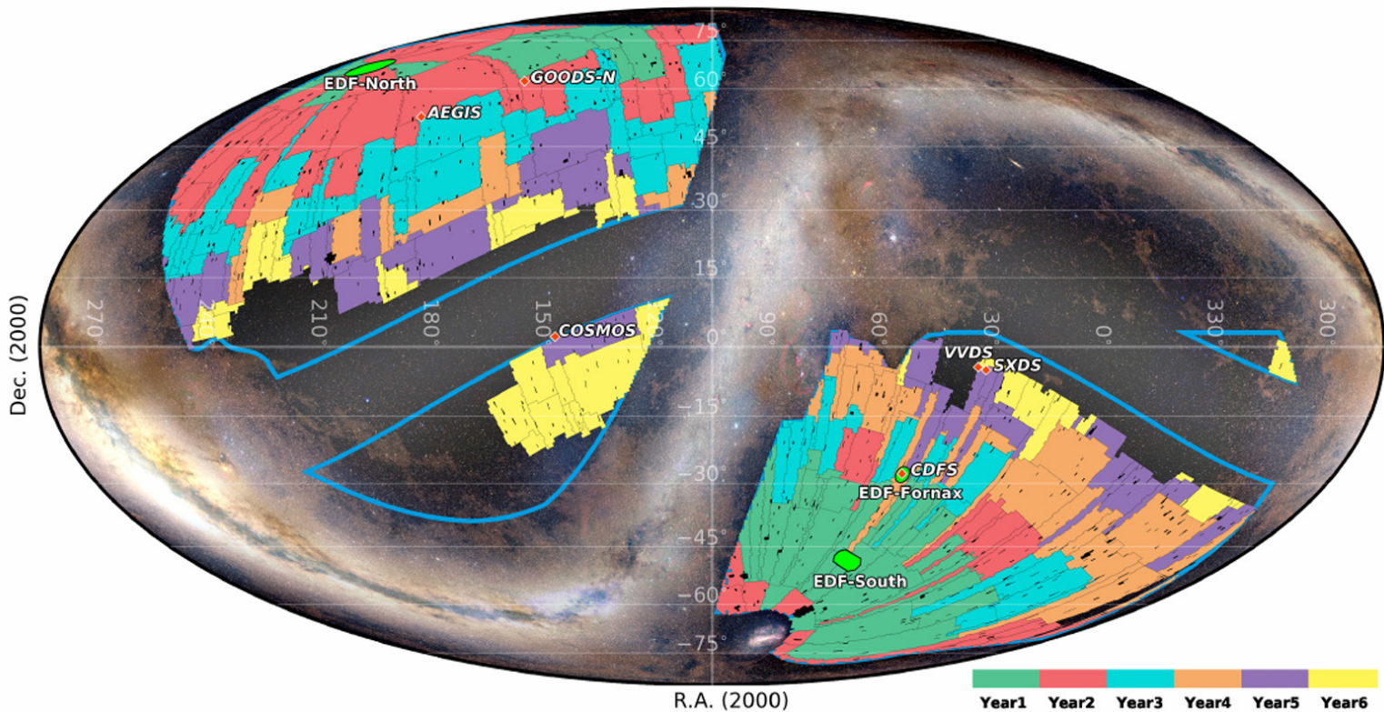
圖2. 歐幾里得巡天計畫，該任務避開銀河盤面及黃道面，框區域涵蓋約16,000平方度，預計觀測約13,416平方度，不同顏色表示不同年份的觀測目標。淺綠色顯示歐幾里得深空巡天計畫，深紅色標示深空巡天的輔助觀測目標（未按比例）。圖片來源： https://arxiv.org/pdf/2405.13491
