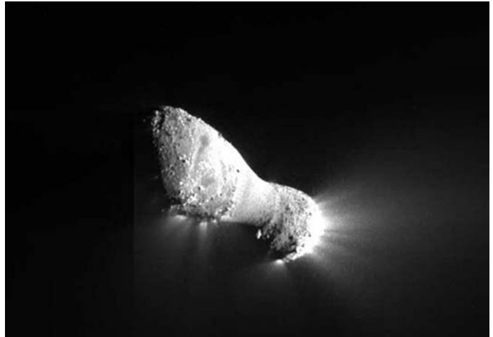
圖10. EPOXI任務所取得的哈特雷2號彗星影像。揭示了彗星表面明顯的冰和塵埃區域，雙葉形狀顯示由兩個主要部分組成。圖片來源：NASA/JPL-Caltech/UMD
