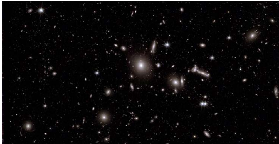
圖7. Abell 2764星系團。
