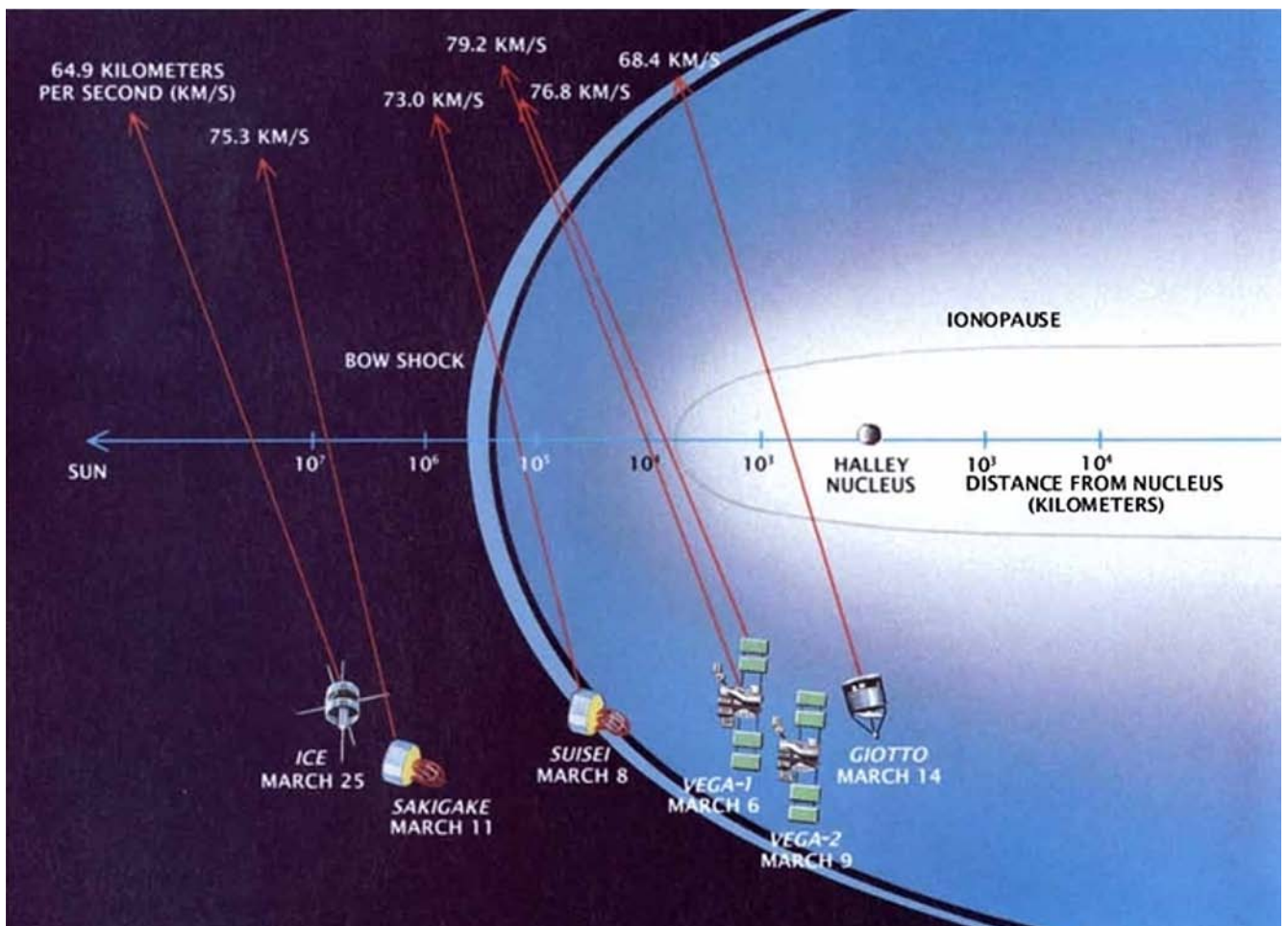
圖4.哈雷艦隊飛掠哈雷彗星。圖片來源：ESA
