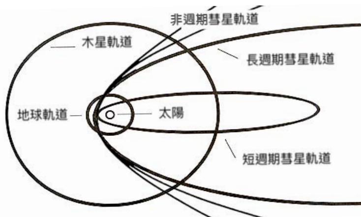
圖1. 彗星軌道示意圖
