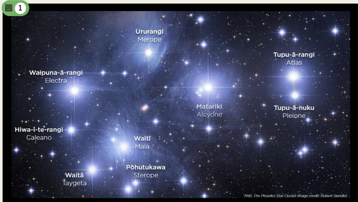
毛利人賦予昴宿星團中恆星的名稱，圖中所示上排是毛利人的名稱，下排是英文的名稱。
