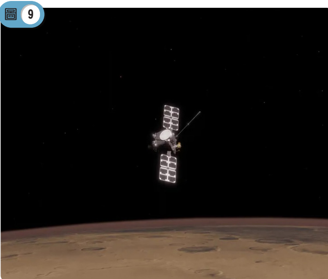
位於環繞火星軌道上的ESCAPADE太空探測器示意圖。圖片來源：NASA
