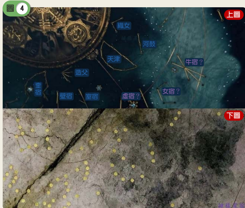
《妖貓傳》劇中穹頂之牛女虛三星宿（上）具有的星形，在龜虎古墳天文圖「復原版」（下）因為剝落而不易辨認。
