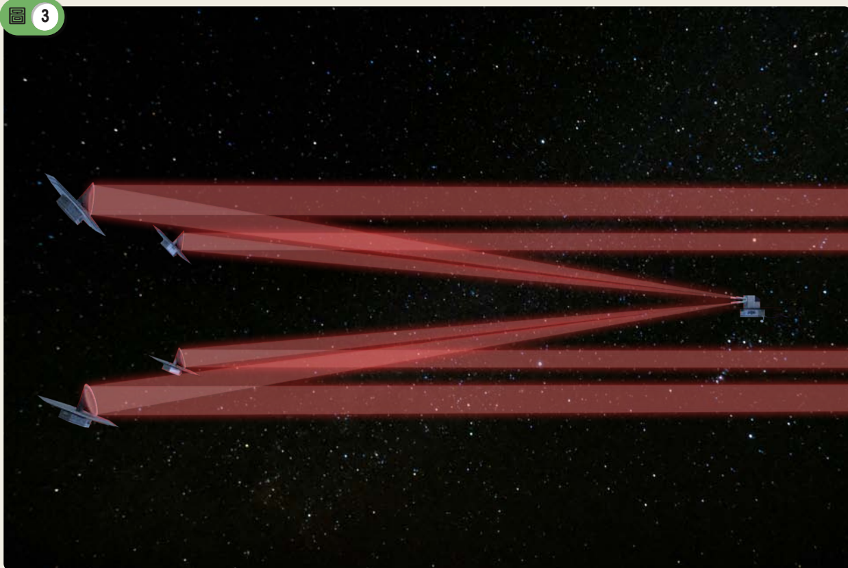
「生命任務」太空望遠鏡是由四個獨立的太空反射鏡與一個光束接收器共同組成，這些望遠鏡將以編隊的方式協同運作，檢測系外行星大氣中的外星生命跡證。圖片來源：LIFE,ETHZurich
