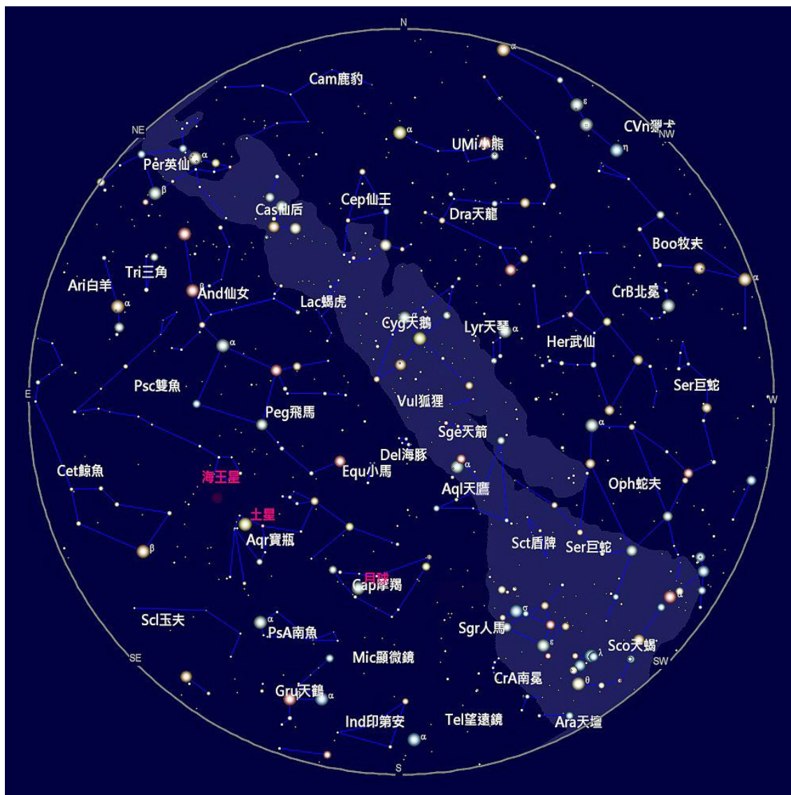
2024 年 9 月 15 日 21:00 的天空
