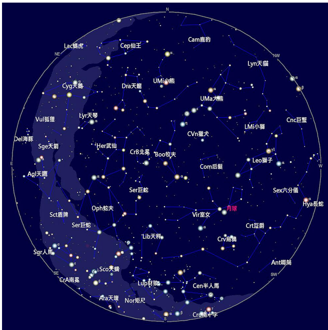
2024 年 6 月 15 日 21:00 的天空
