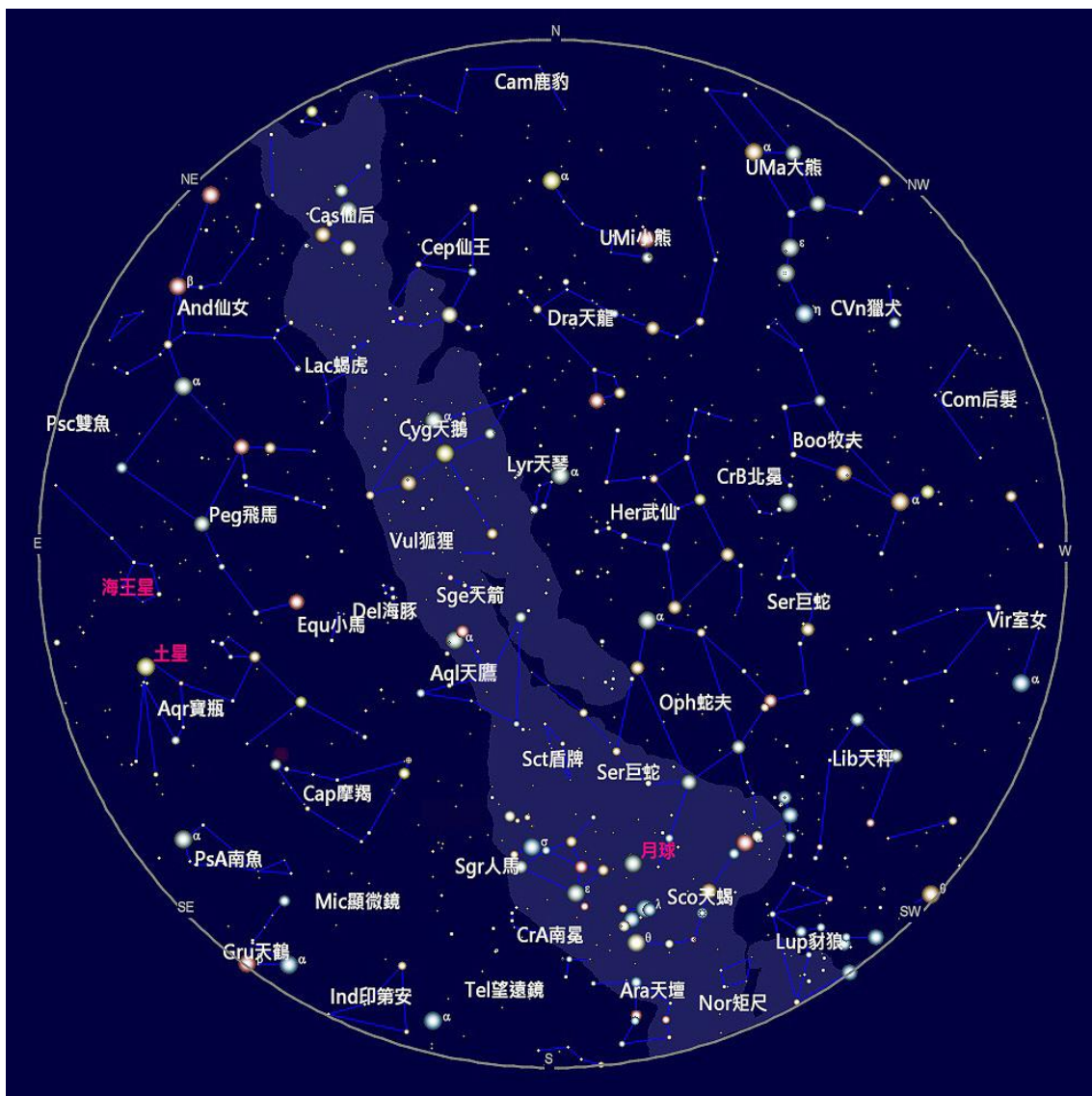
2024 年 8 月 15 日 21:00 的天空
