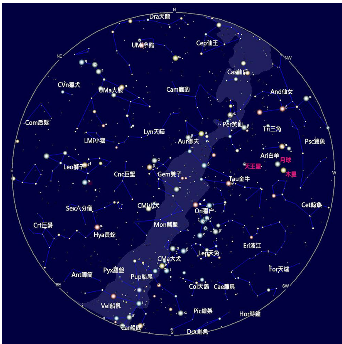
2024 年 2 月 15 日 21:00 的天空
