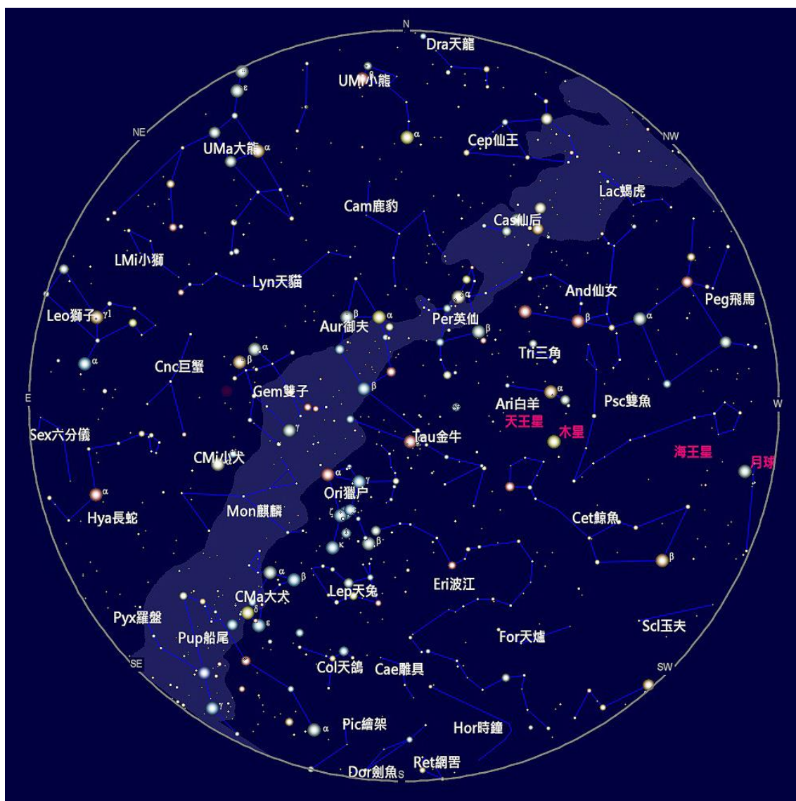
2024 年 1 月 15 日 21:00 的天空
