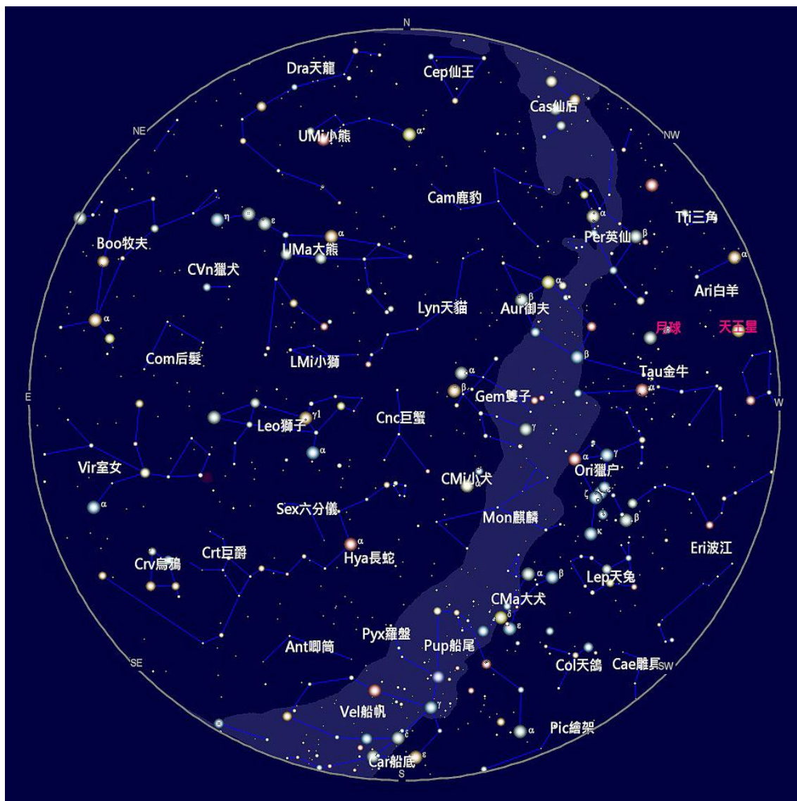
2024 年 3 月 15 日 21:00 的天空
