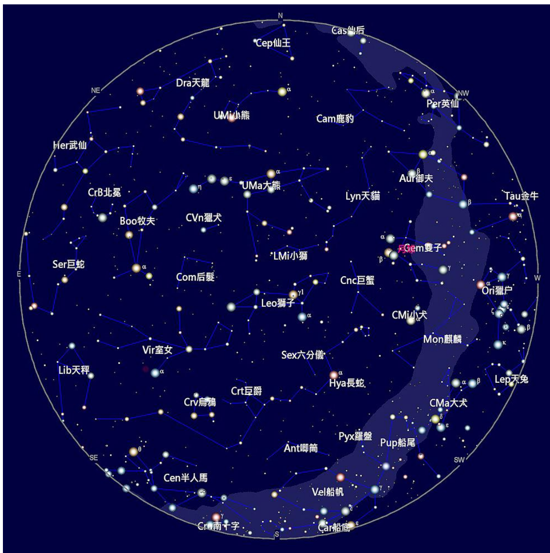
2024 年 4 月 15 日 21:00 的天空
