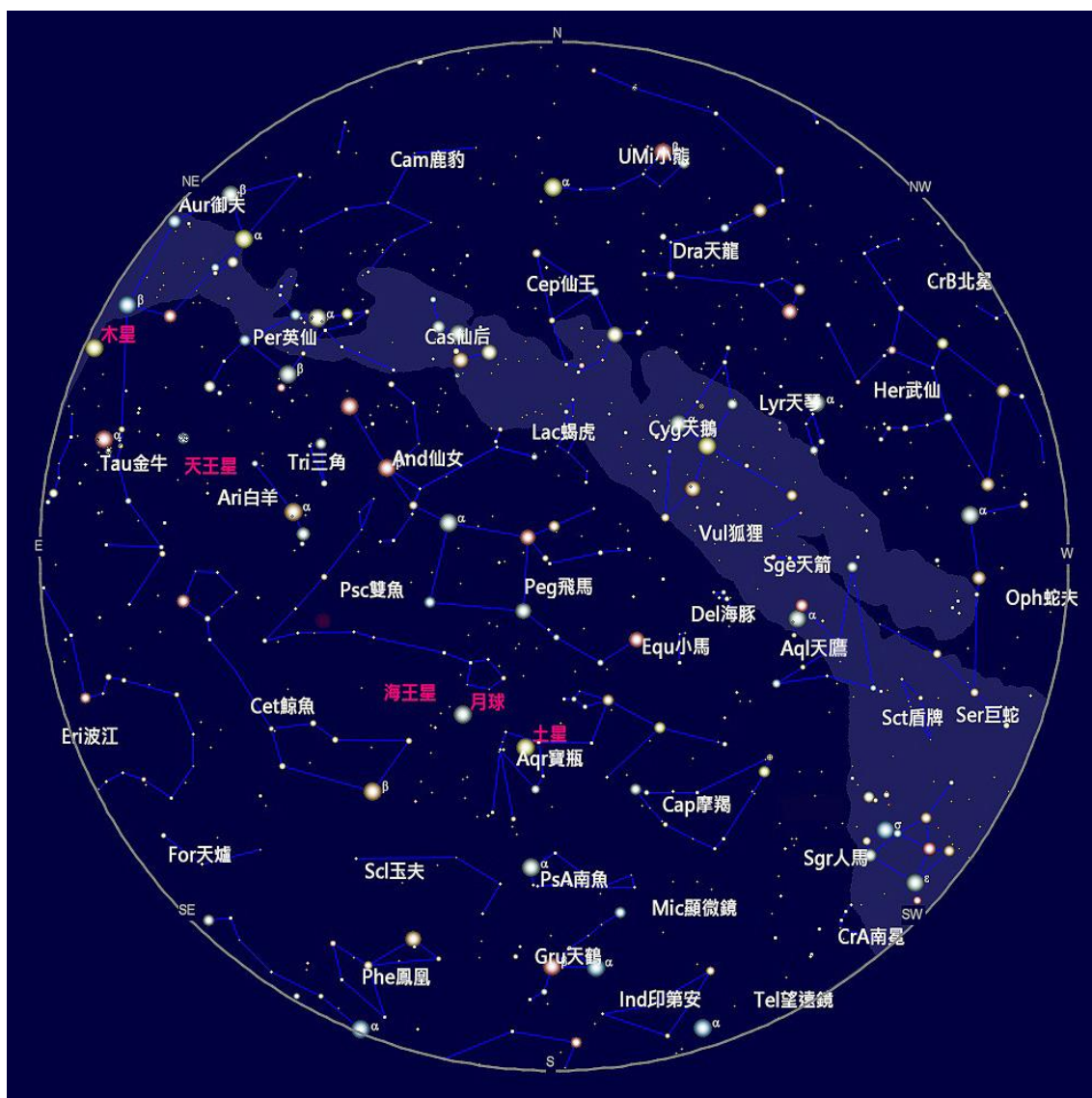
2024 年 10 月 15 日 21:00 的天空
