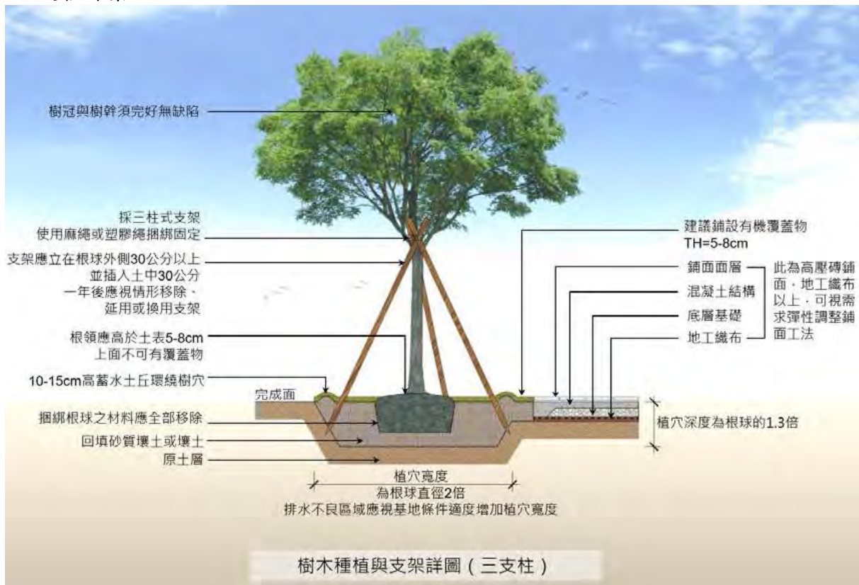
圖 13 喬木類移植施工剖面圖
