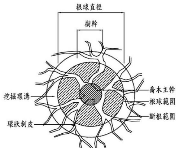
圖 9 喬木斷根平面圖
