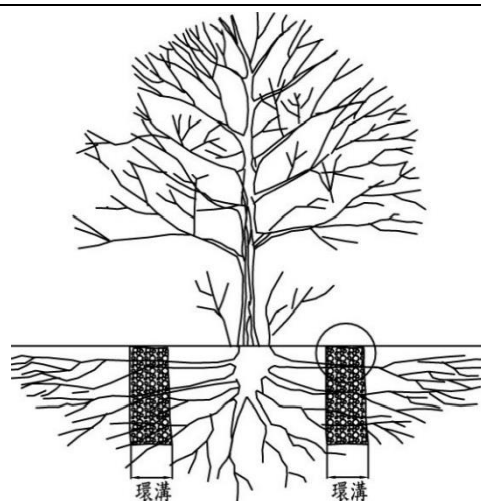
圖 10 喬木斷根剖面圖
