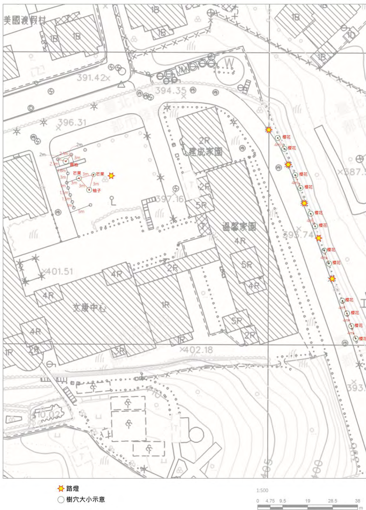
圖 4 定植平面配置圖
