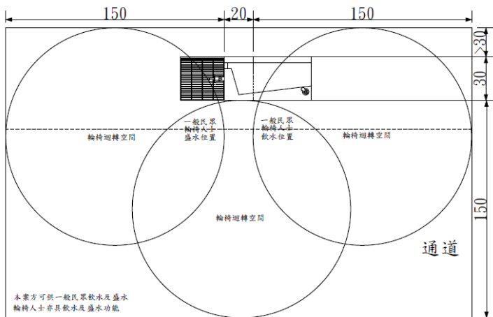
上視圖
