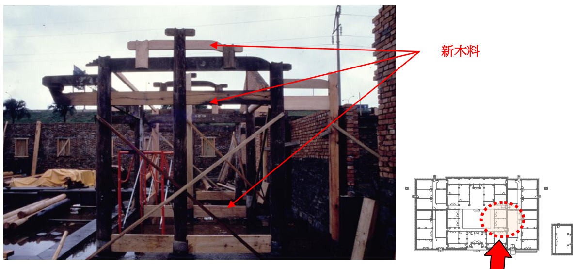
【圖 3-121】「東廂房」重組時屋架之新木料位置 資料來源：重耀建築師事務所提供
