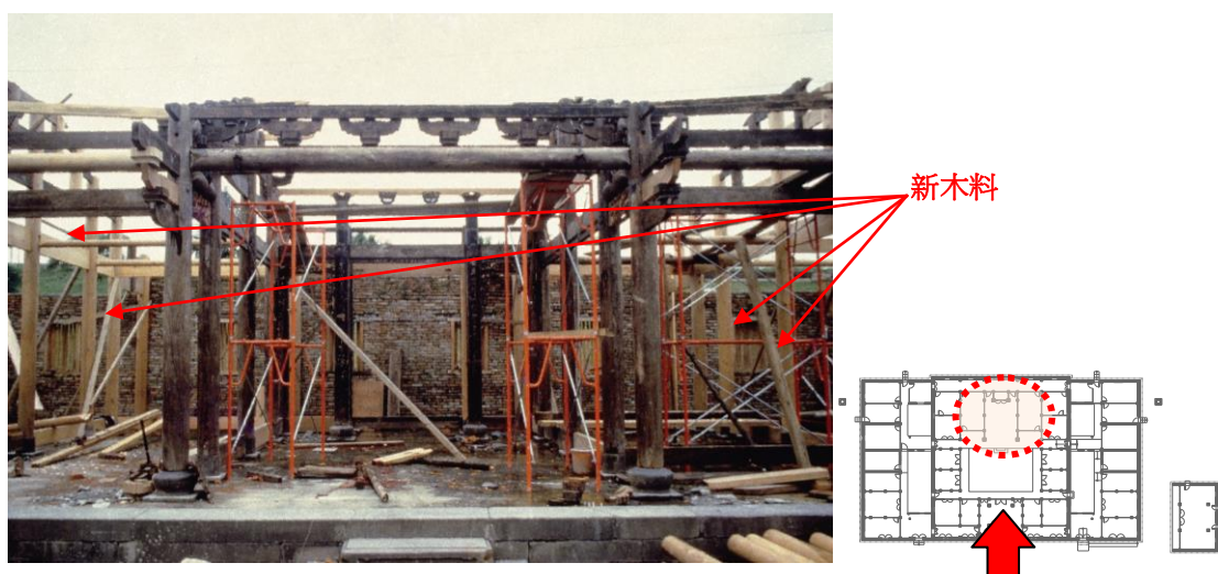
【圖 3-123】「正廳、大房、二房」重組時木柱、桁樑之新木料位置， 可以發現正廳兩邊之大房與二房更新之木料佔多數。 資料來源：重耀建築師事務所提供
