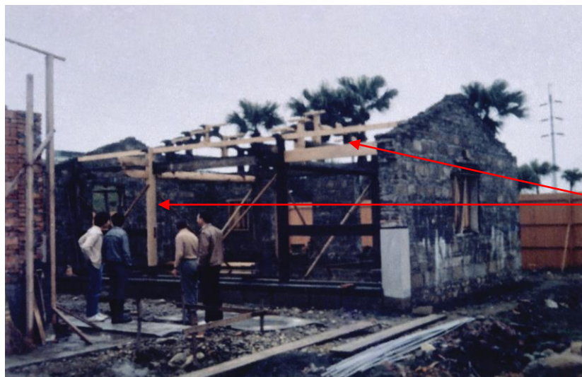
【圖 3-118】「書房」重組時屋架之新木料位置。
