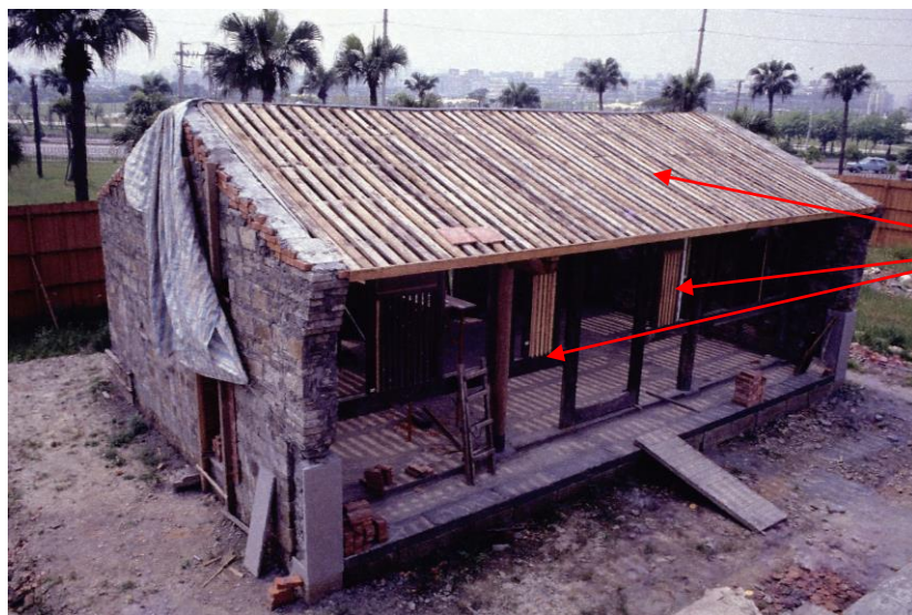
【圖 3-119】「書房」重組時屋頂椽條已全面更新。
