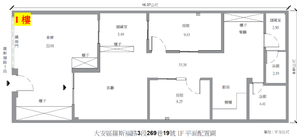
平面配置圖
