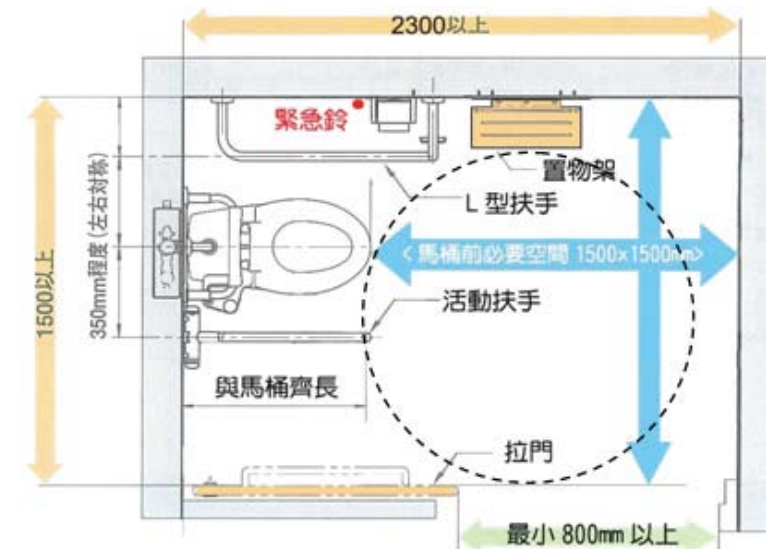
無障礙廁所相關設施（平面圖）
