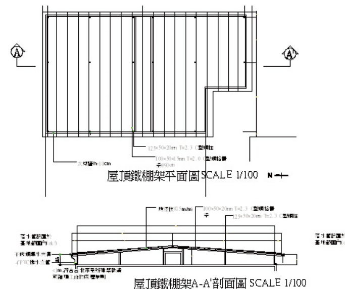
屋頂鐵棚架竣工平、剖面圖
