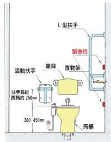
無障礙廁所相關設施（立面圖）
