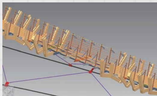
▲ 施作前，精密運算下的橋身3D模擬圖。
