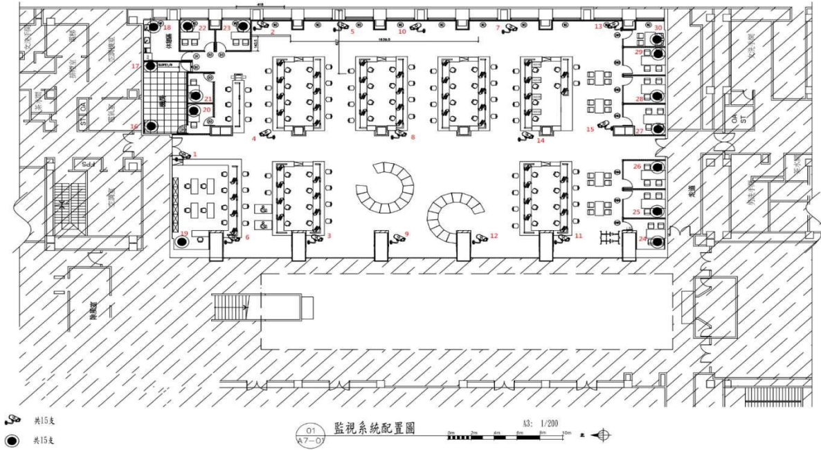
北區聯合服務中心監視系統配置圖
