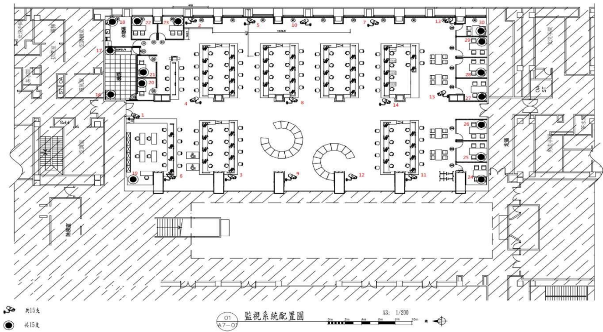
北區聯合服務中心監視系統配置圖
