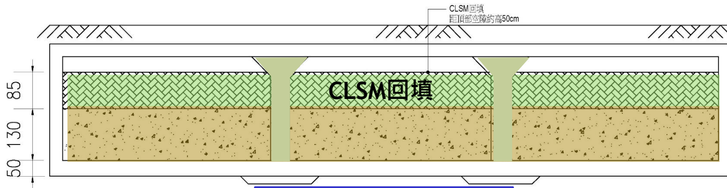
CLSM回填剖面圖
