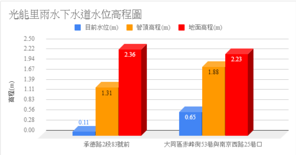
圖3.8 光能里雨水下水道水位高程圖
