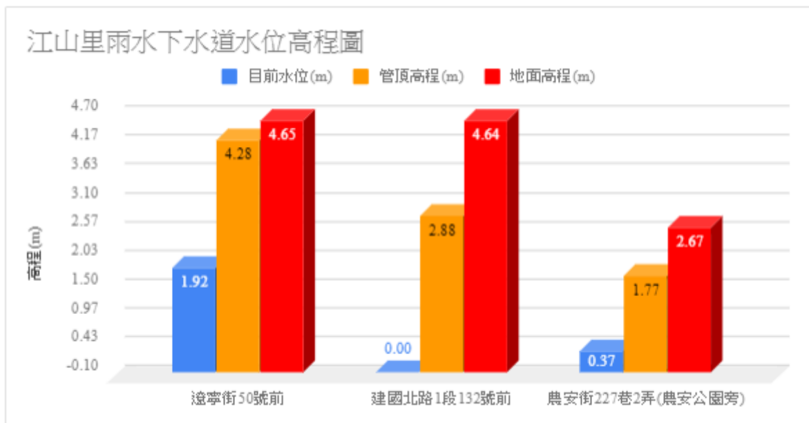
圖3.8 江山里雨水下水道水位高程
