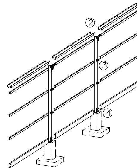
VBP 溫室側面構造組立示意圖(B)
