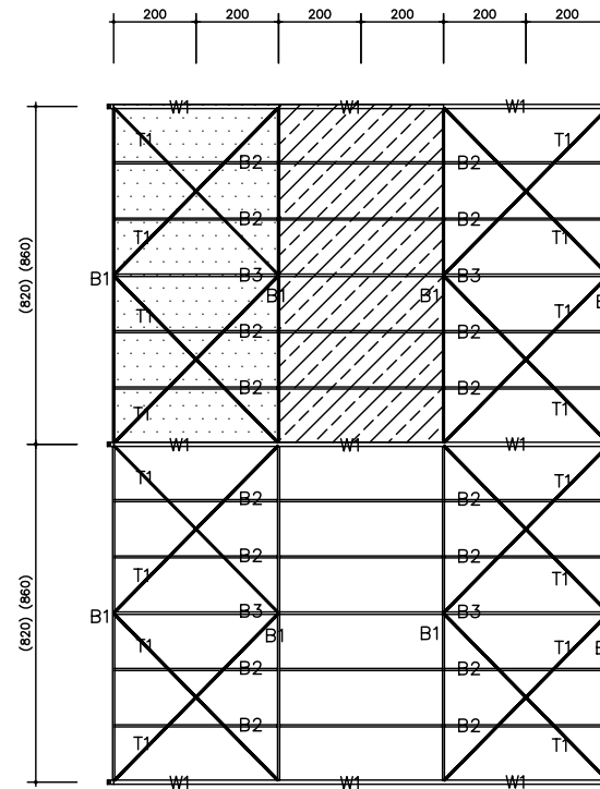
屋頂結構平面圖(2X3單元)
