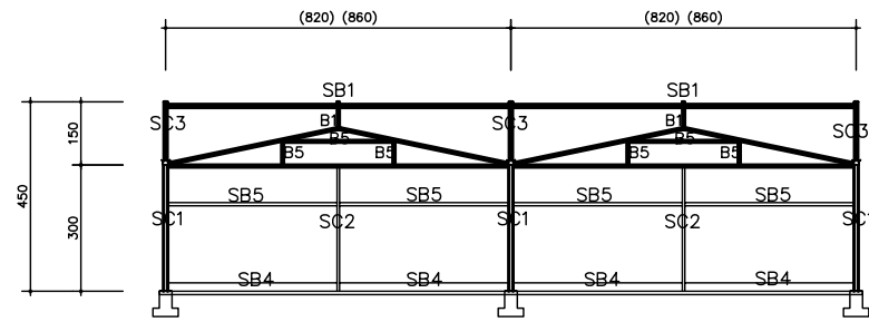
背立面圖(2X3單元)
