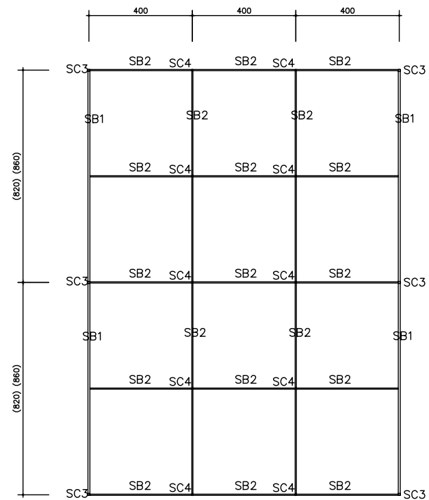
外網架平面圖(2X3單元)
