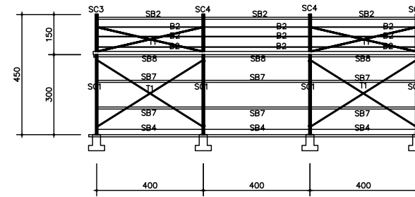
橫剖面圖(2X3單元)
