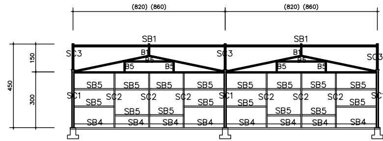
正立面圖(2X3單元)
