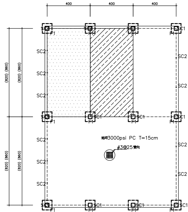
基礎平面圖(2X3單元)
