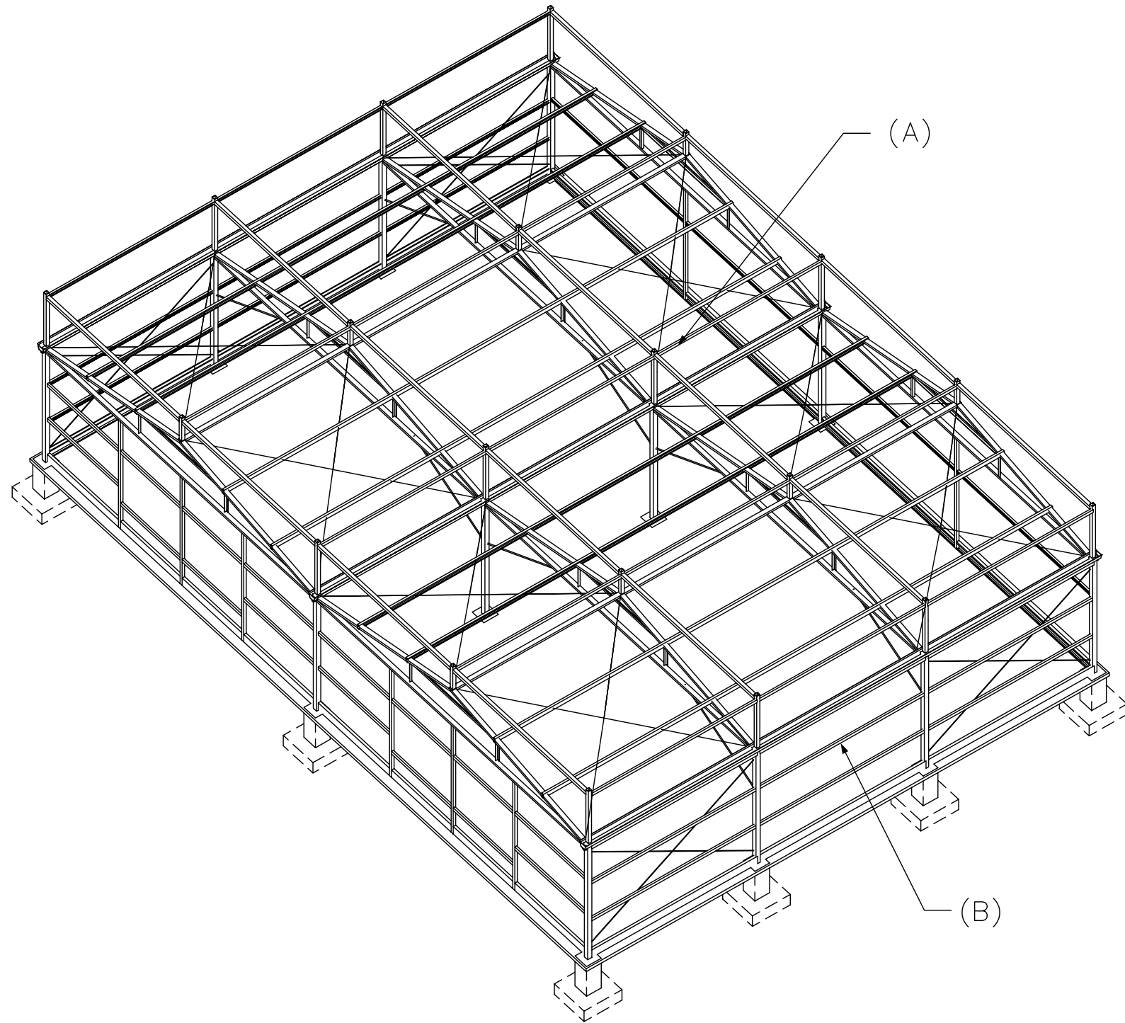
VBP 溫室3單元組立透視示意圖
