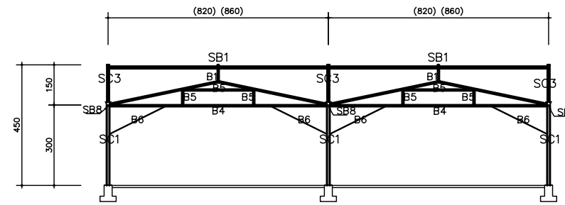
橫剖面圖(2X3單元)
