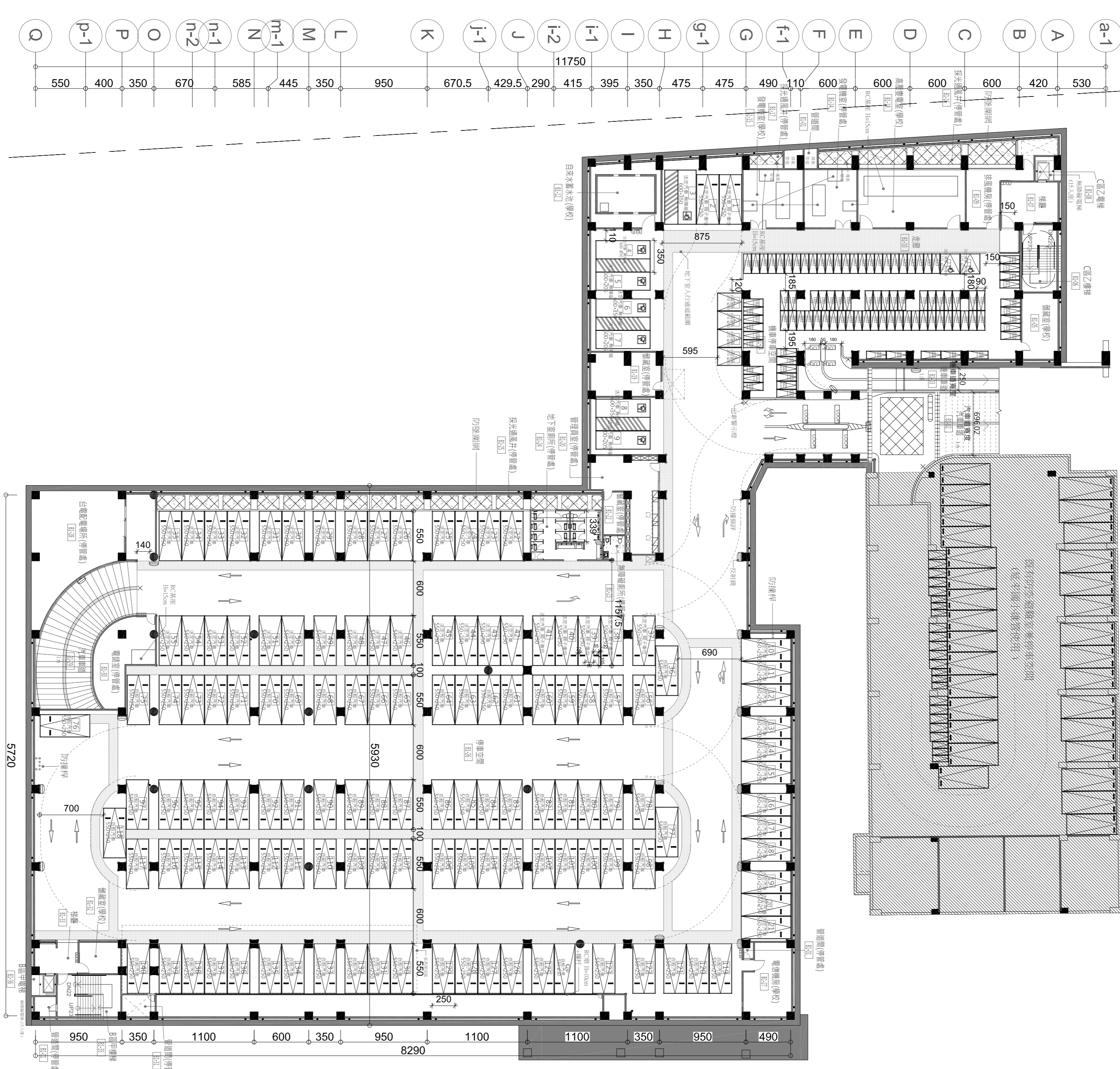
1 地下一層平面圖 A2-02 A1:1:300
