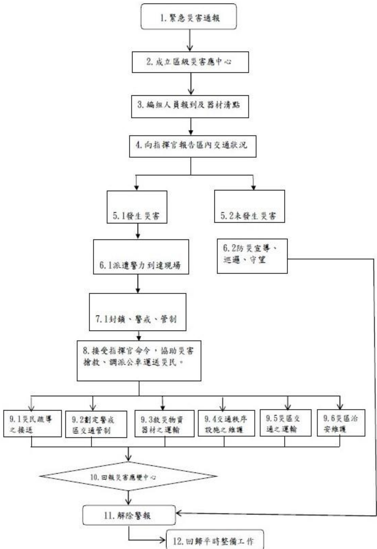
(五)臺北市區災害應變中心交通組標準作業程序圖
