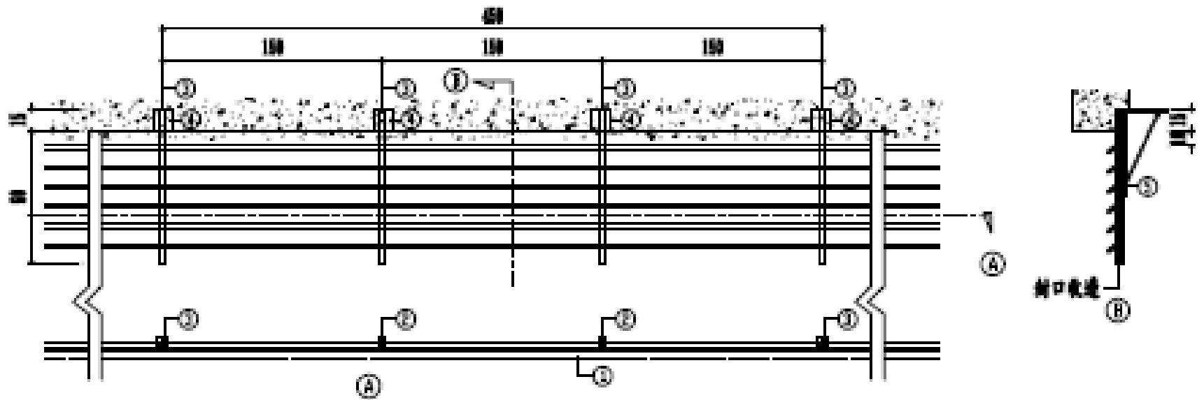
鋁格柵垂直遮陽板詳圖
