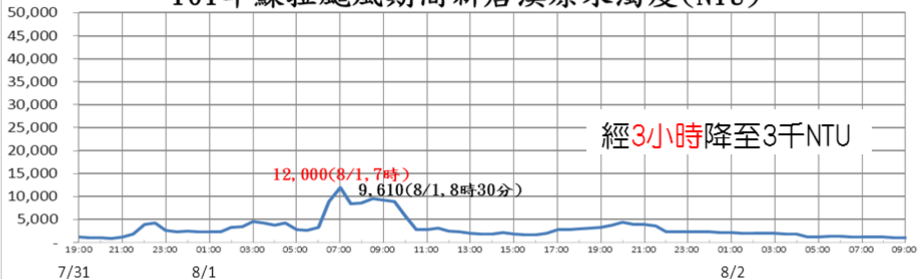
101年蘇拉颱風期間新店溪原水濁度(NTU)
