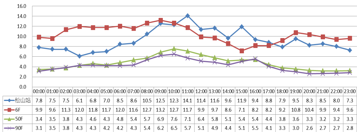
2016/8/5-2016/8/15逐時平均值
