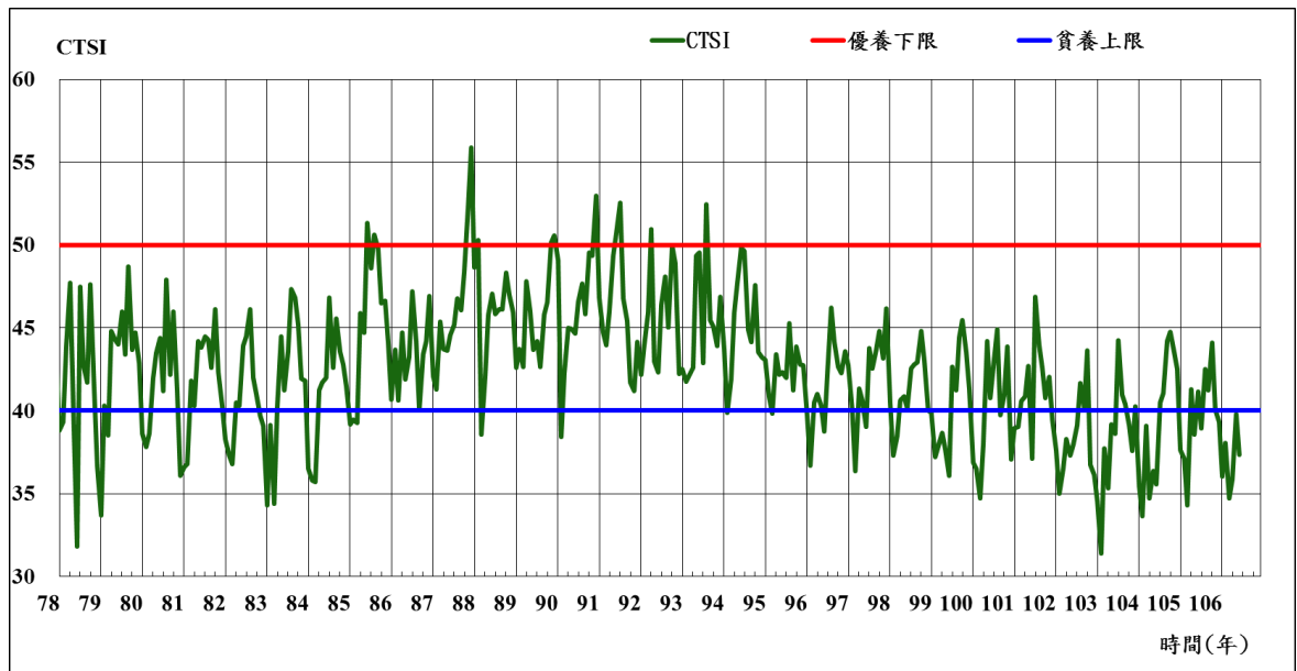
圖 2：翡翠水庫歷年卡爾森優養指數統計圖
