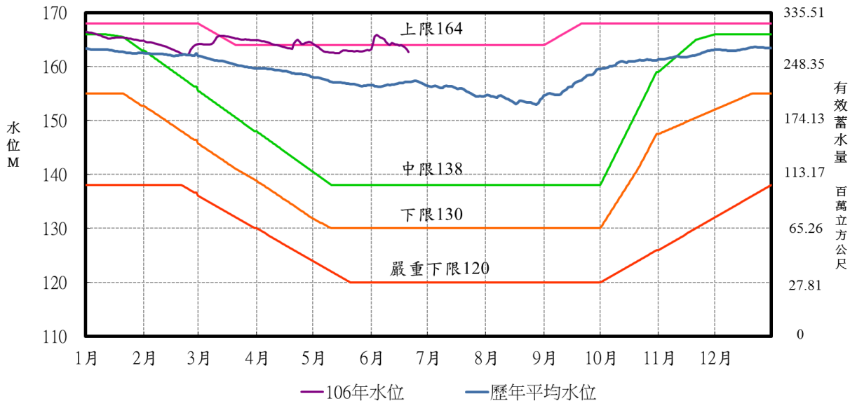
圖 1：106 年翡翠水庫水位歷線圖
