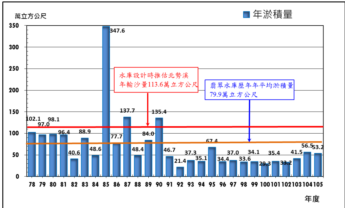
圖 3：翡翠水庫歷年淤積量統計圖
