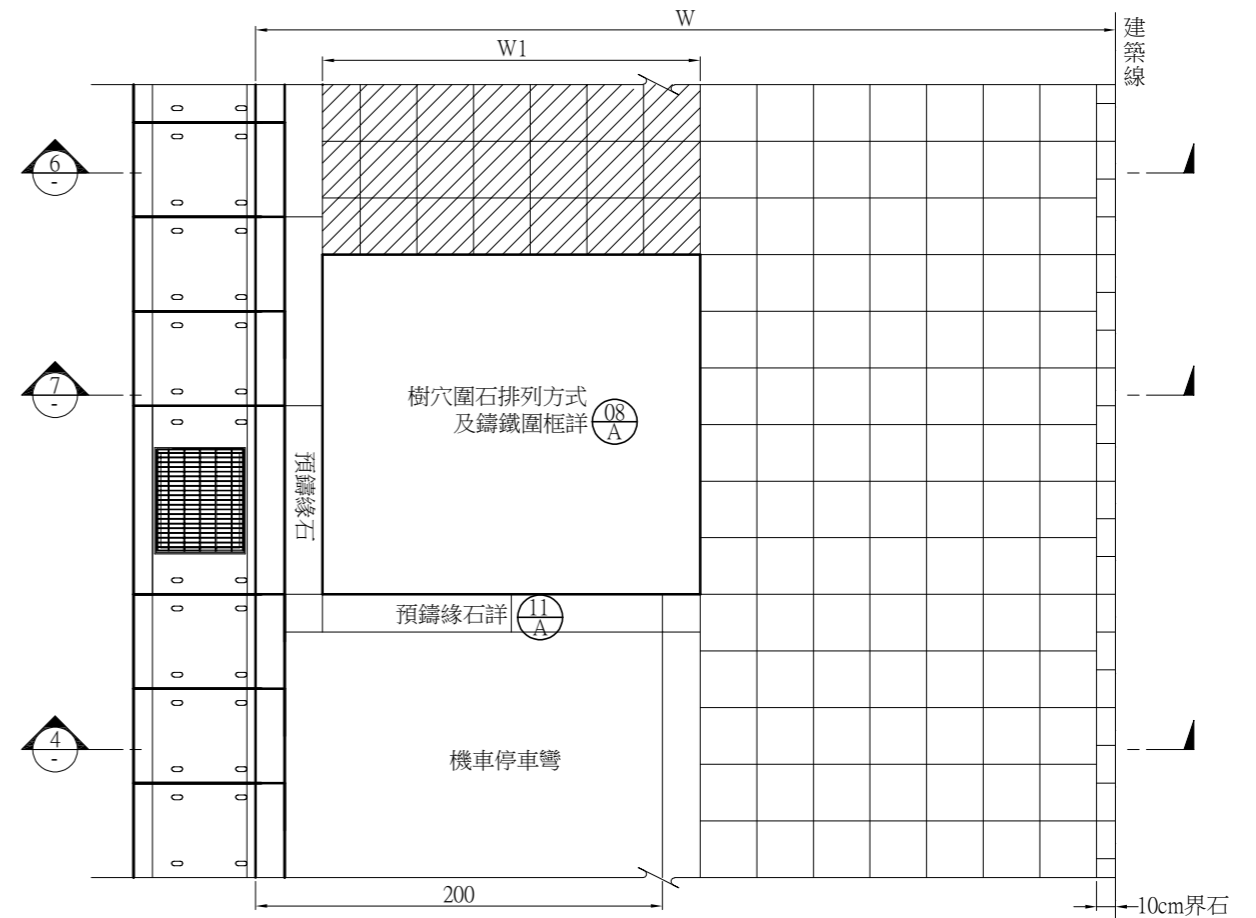
D型鋪面鋪設平面圖
