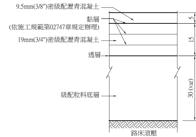
道路斷面參考詳圖 A1 (1:5) A3 (1:10) Unit:cm
