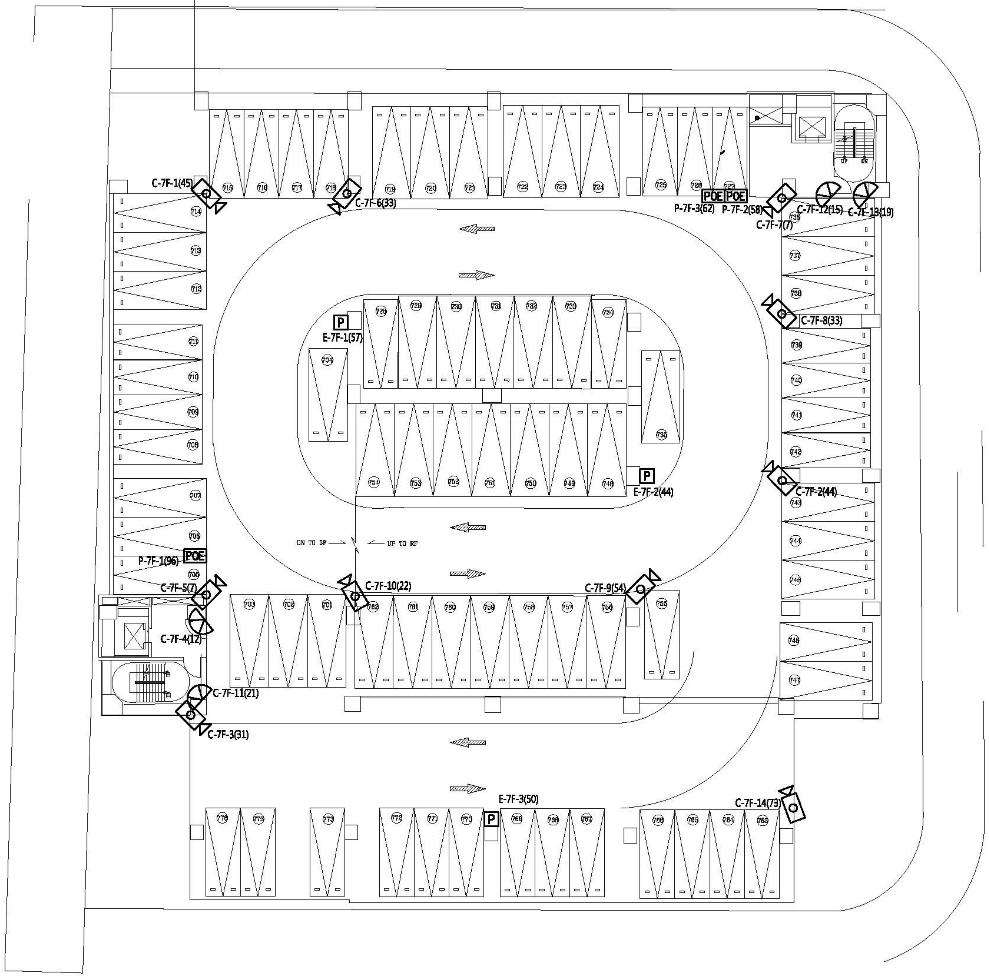
七層平面圖
