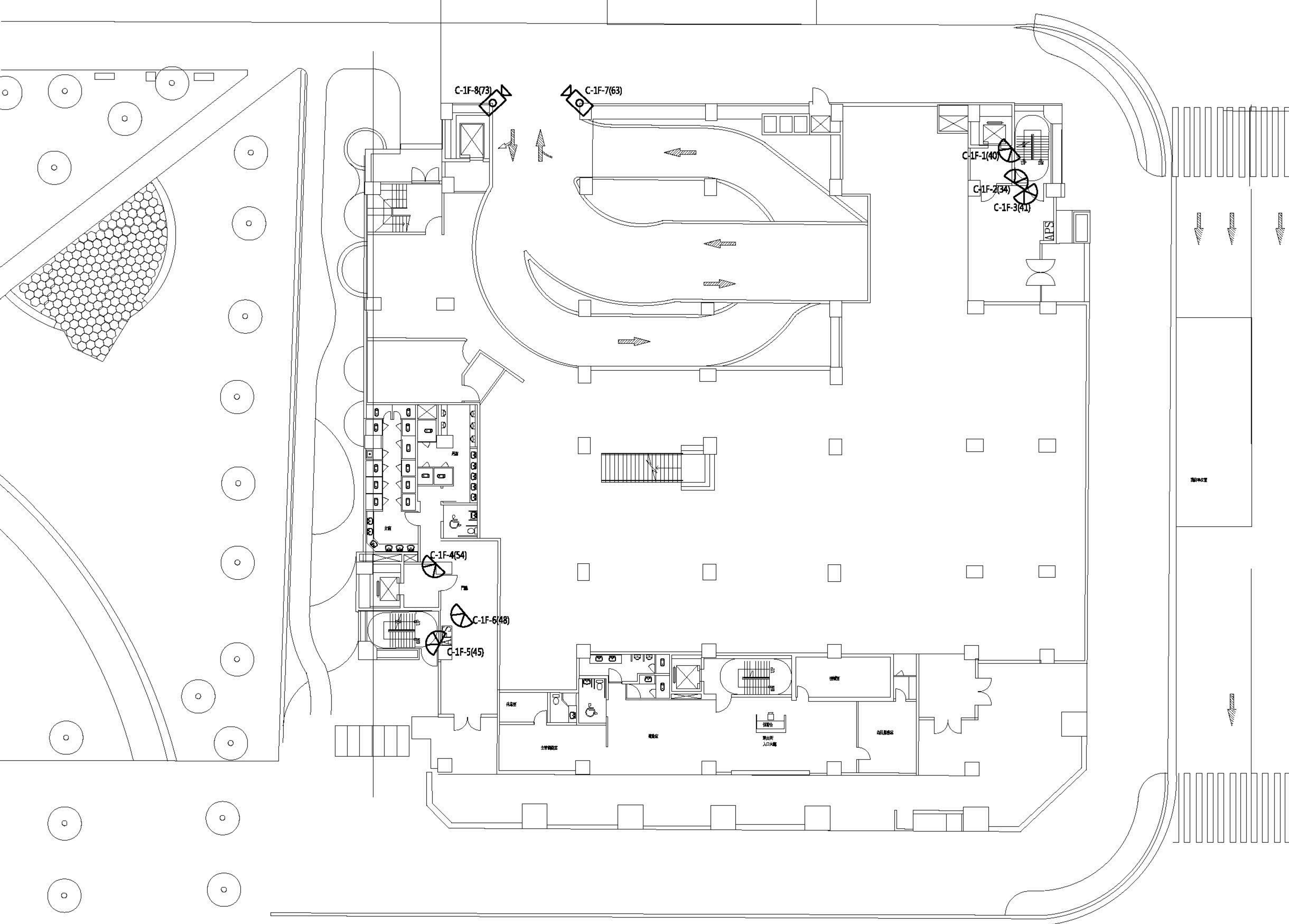
一層平面圖
