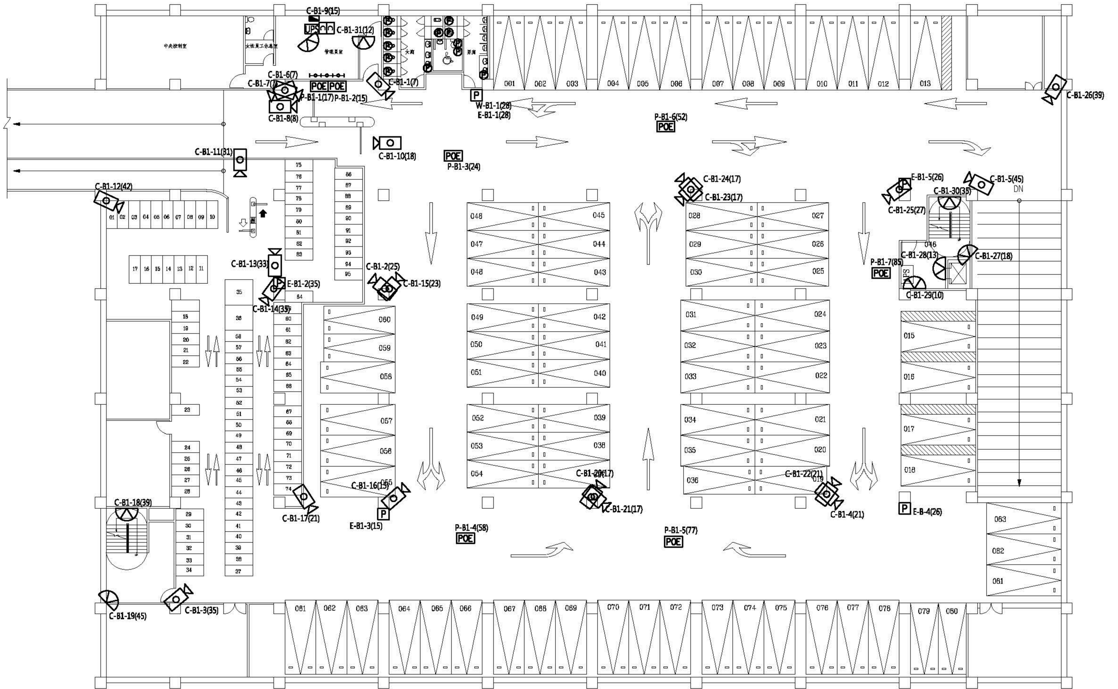
地下一層平面圖
