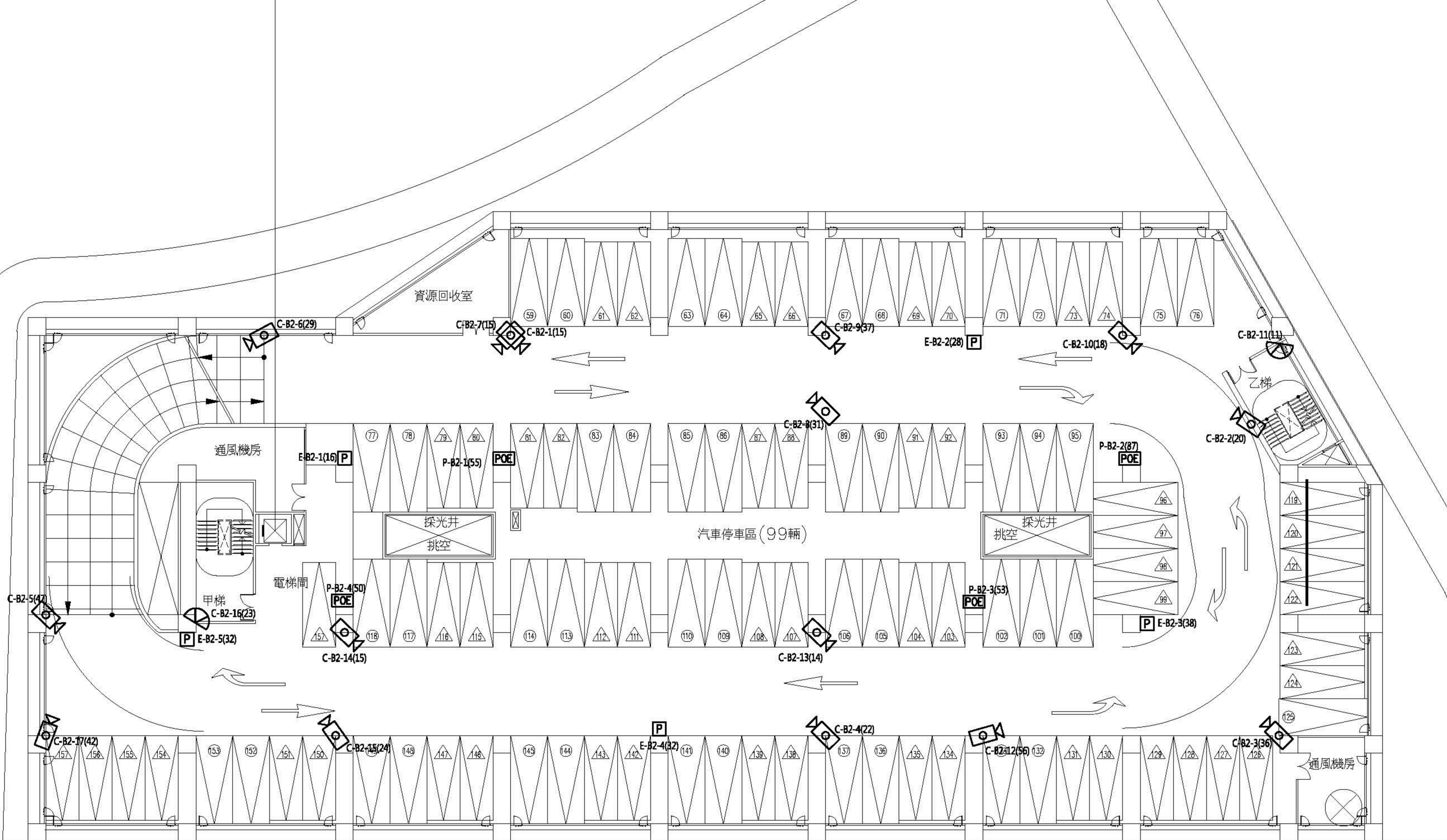
地下二層平面圖
