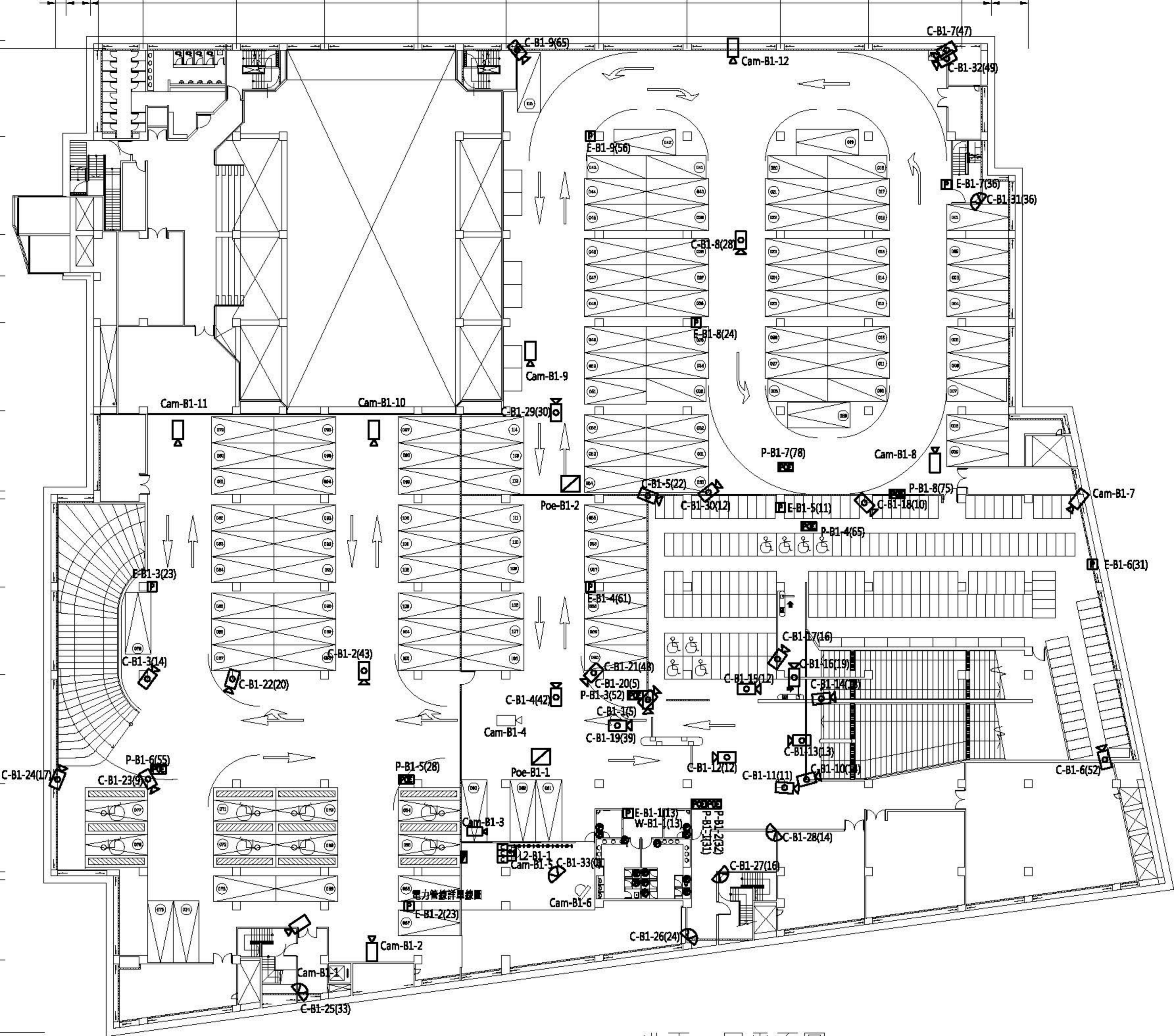
地下一層平面圖
