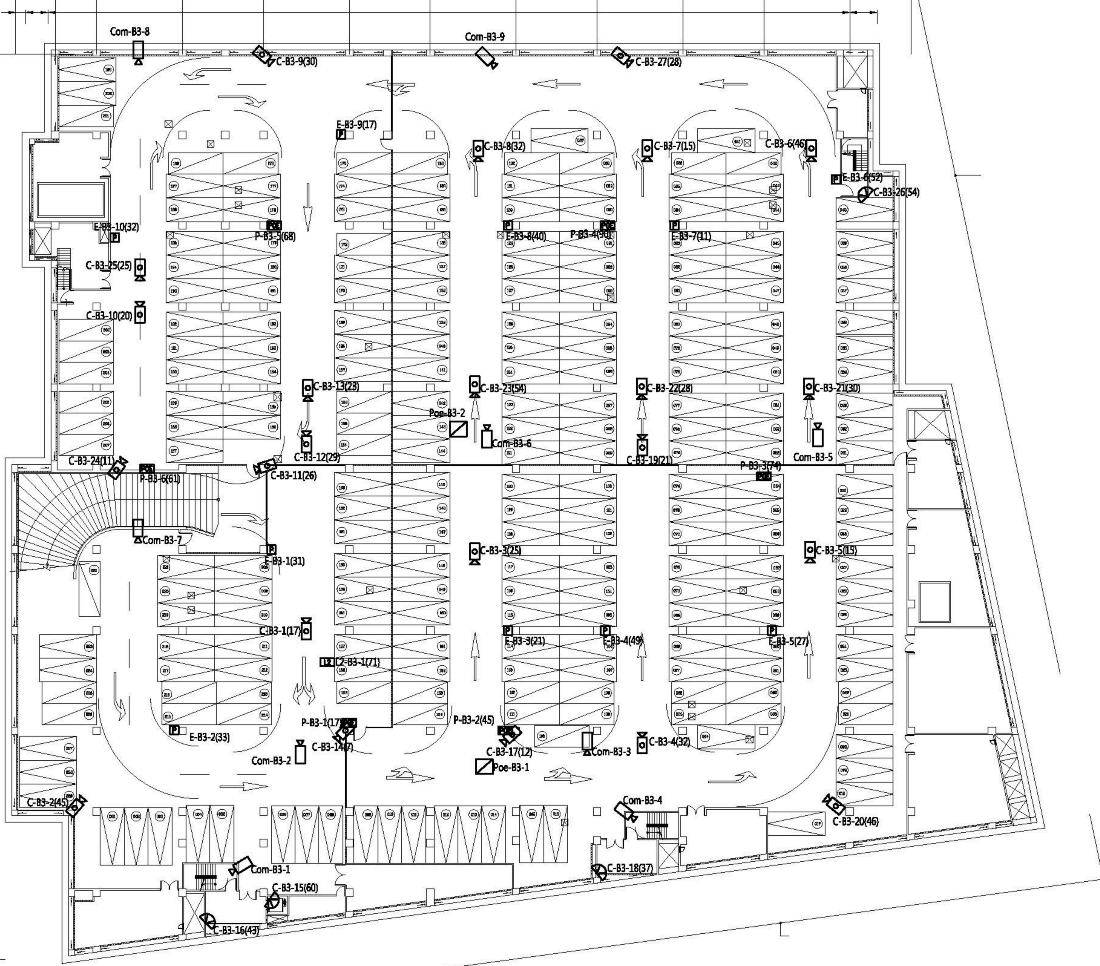
地下三層平面圖
