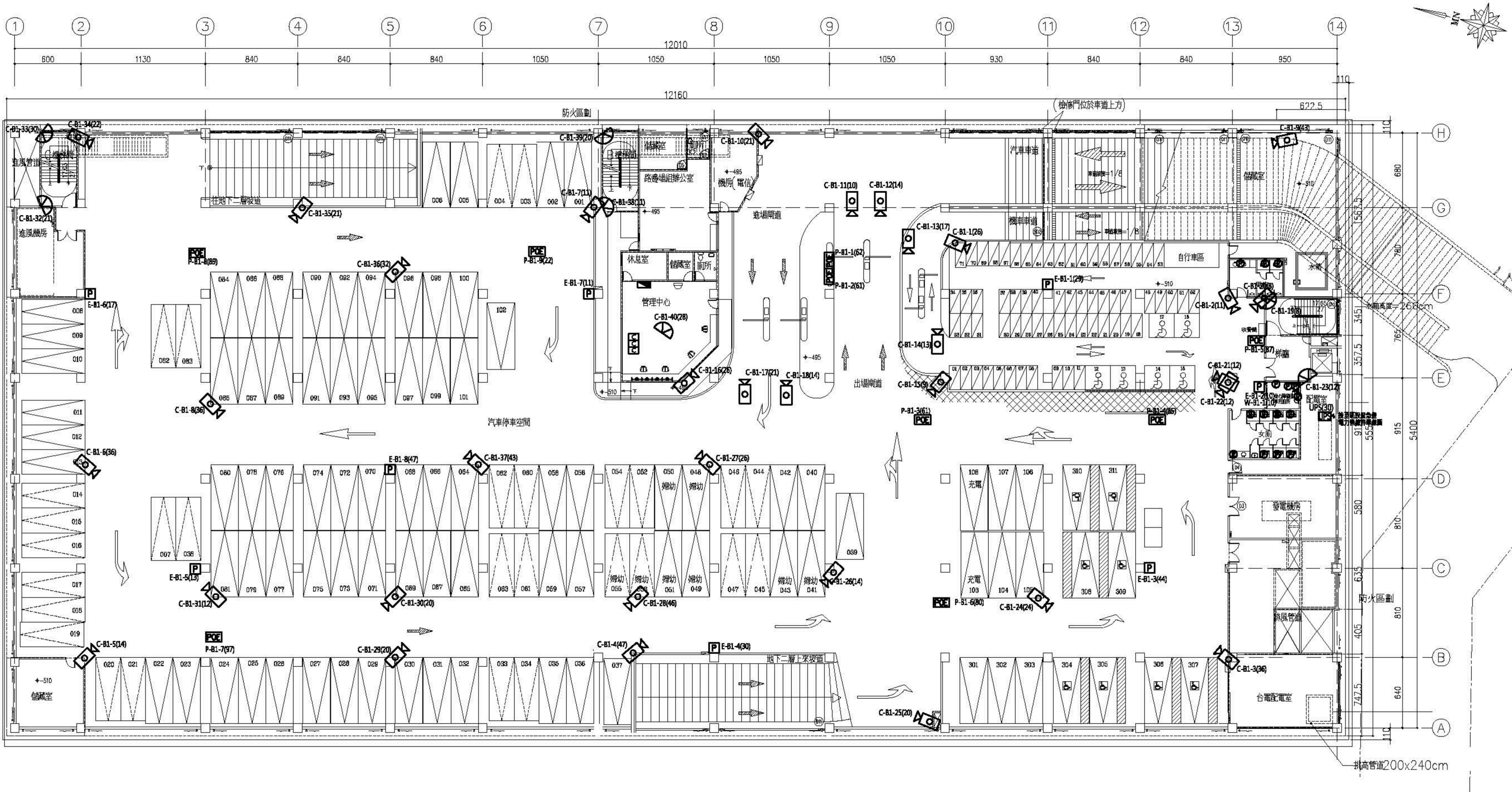
地下一層平面圖
