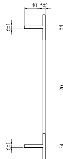
框座剖面圖 A1 (1:2) A3 (1:4) Unit:mm = 4
