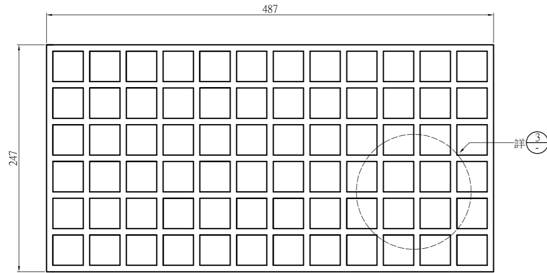
格柵蓋板平面圖 A1 (1:2) A3 (1:4) Unit:mm = 1
