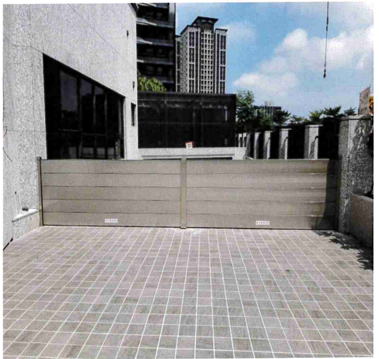
車道組合式防水閘門
