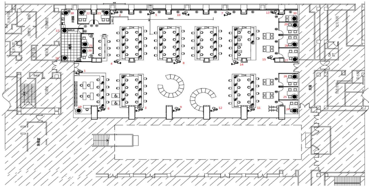
北區聯合服務中心監視系統配置圖
