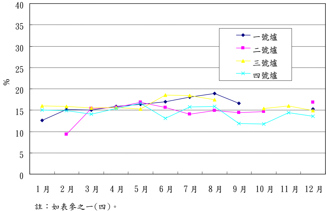
圖參之一(四)8 木柵廠 94 年含水率容積比排放監測值
