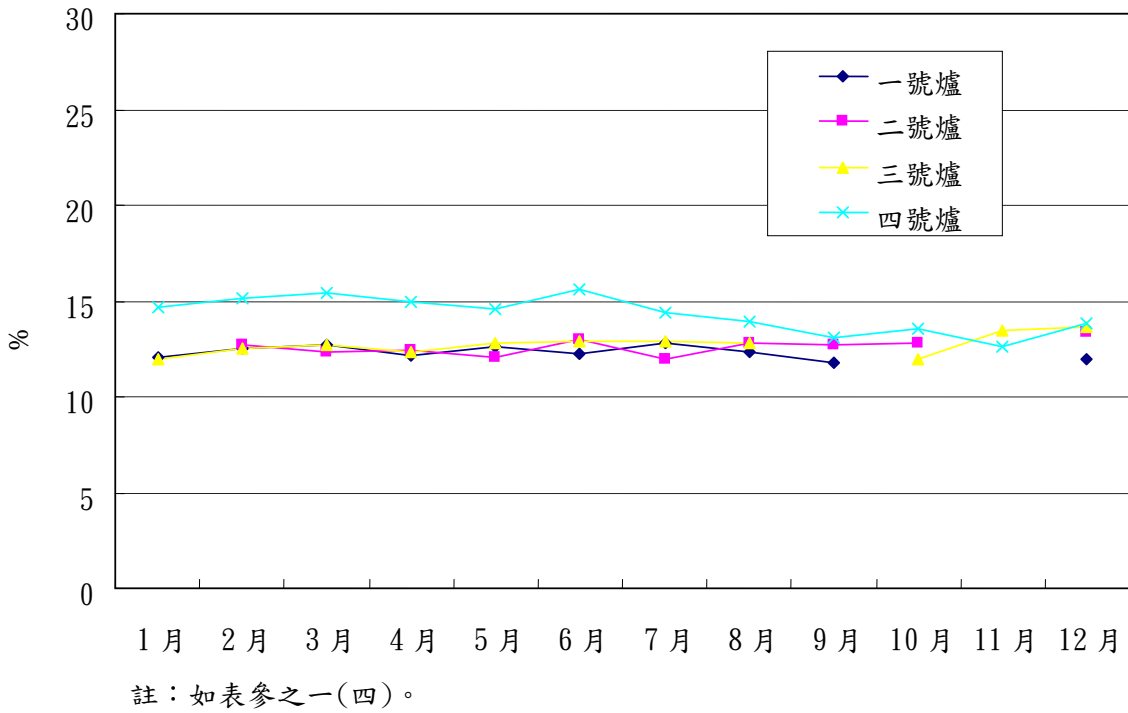
圖參之一(四)7 木柵廠 94 年含氧率容積比排放監測值
