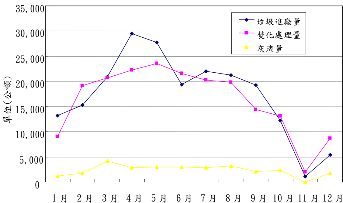
圖貳之一 木柵廠 94 年焚化操作營運統計圖
