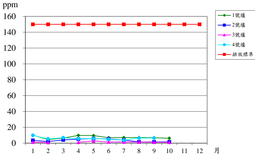
圖參之一(二)-5-112 年一氧化碳(CO)排放監測值
