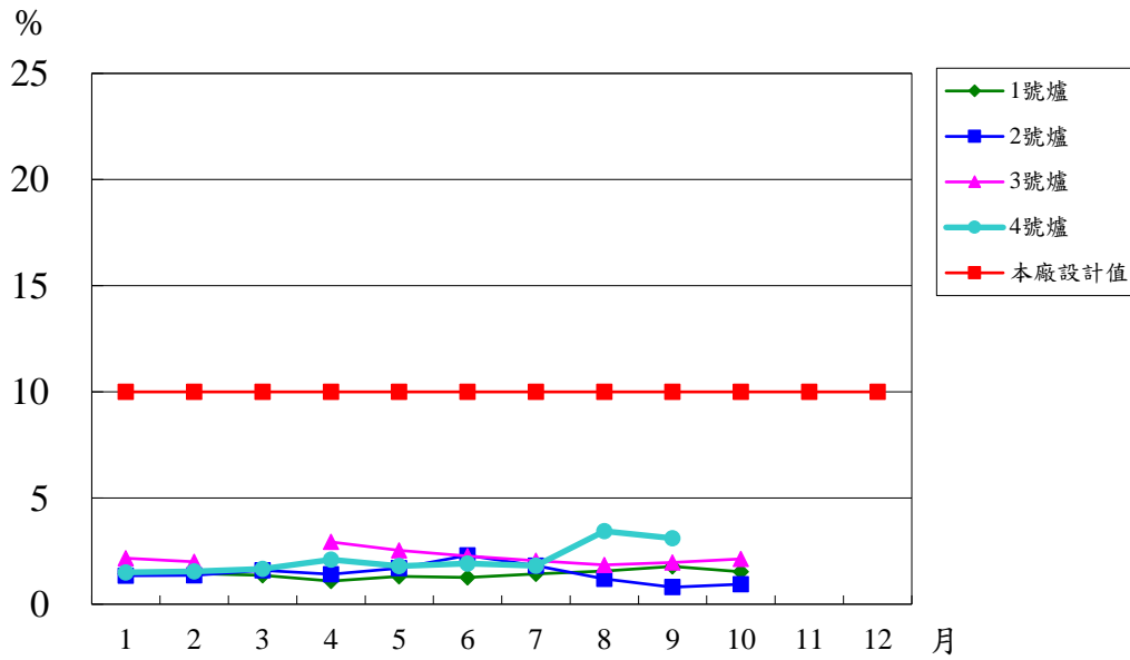
圖參之一(二)-7-112 年含氧率排放監測值
