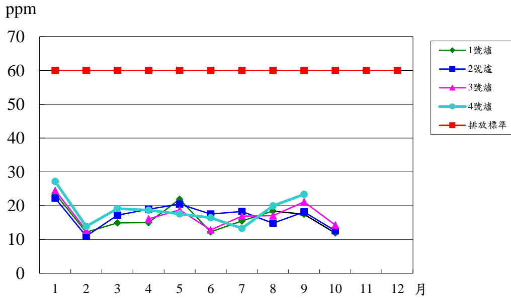
圖參之一(二)-3-112 年氮氧化物(NOx)排放監測值
