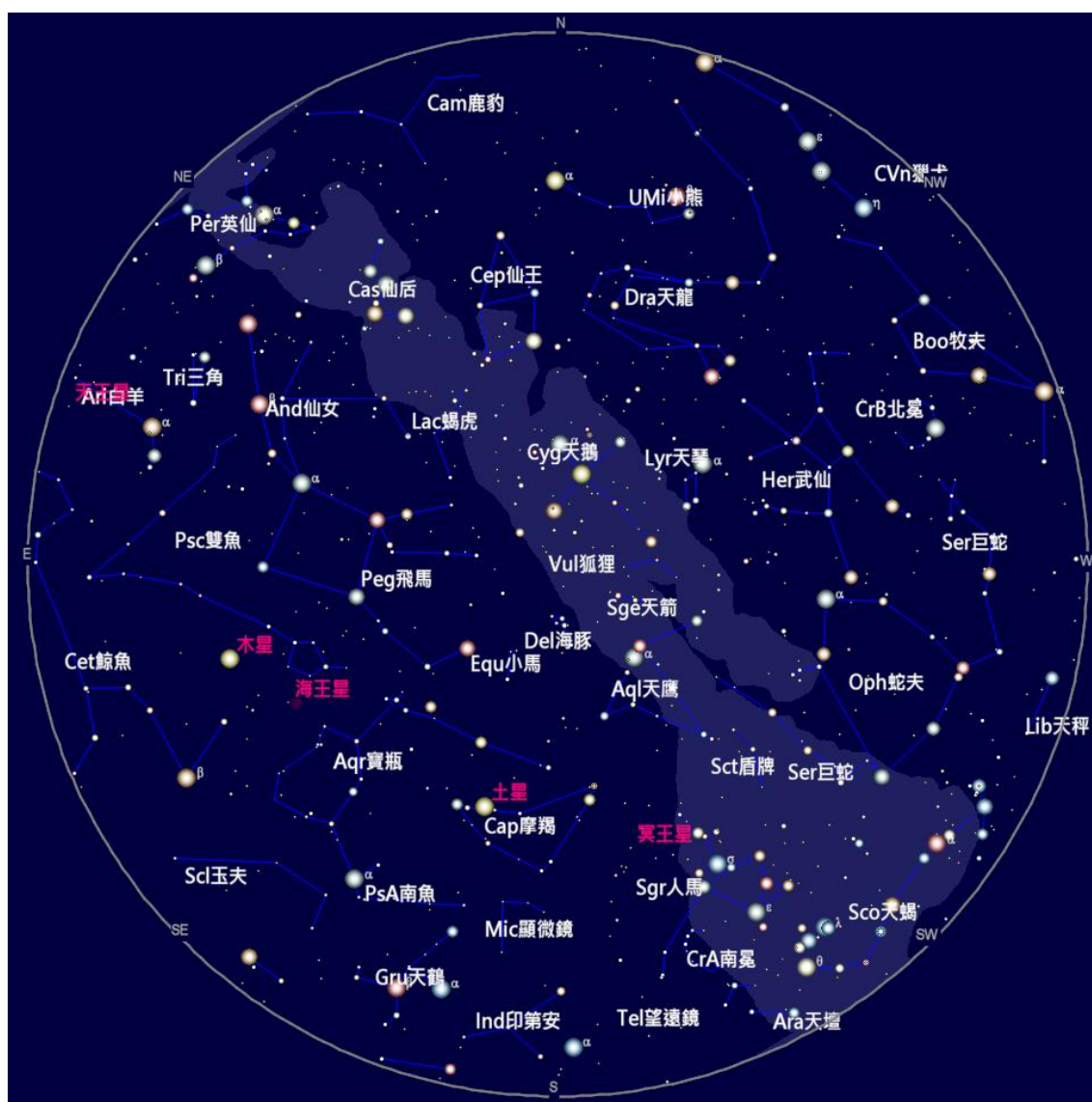
2022 年 9 月 15 日 21:00 的天空
