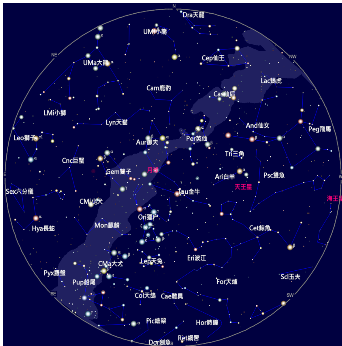
2022 年 1 月 15 日 21:00 的天空
