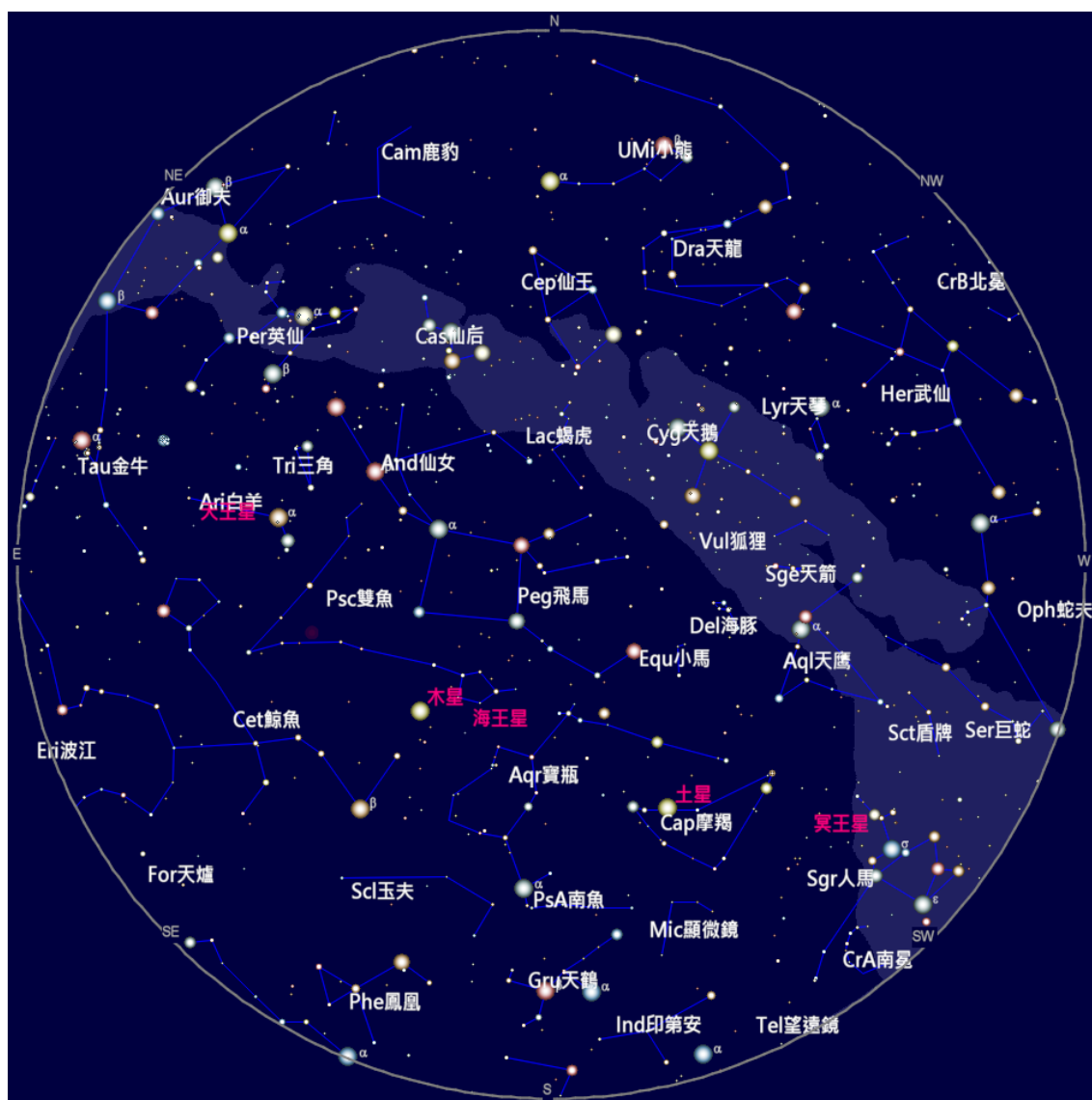
2022 年 10 月 15 日 21:00 的天空
