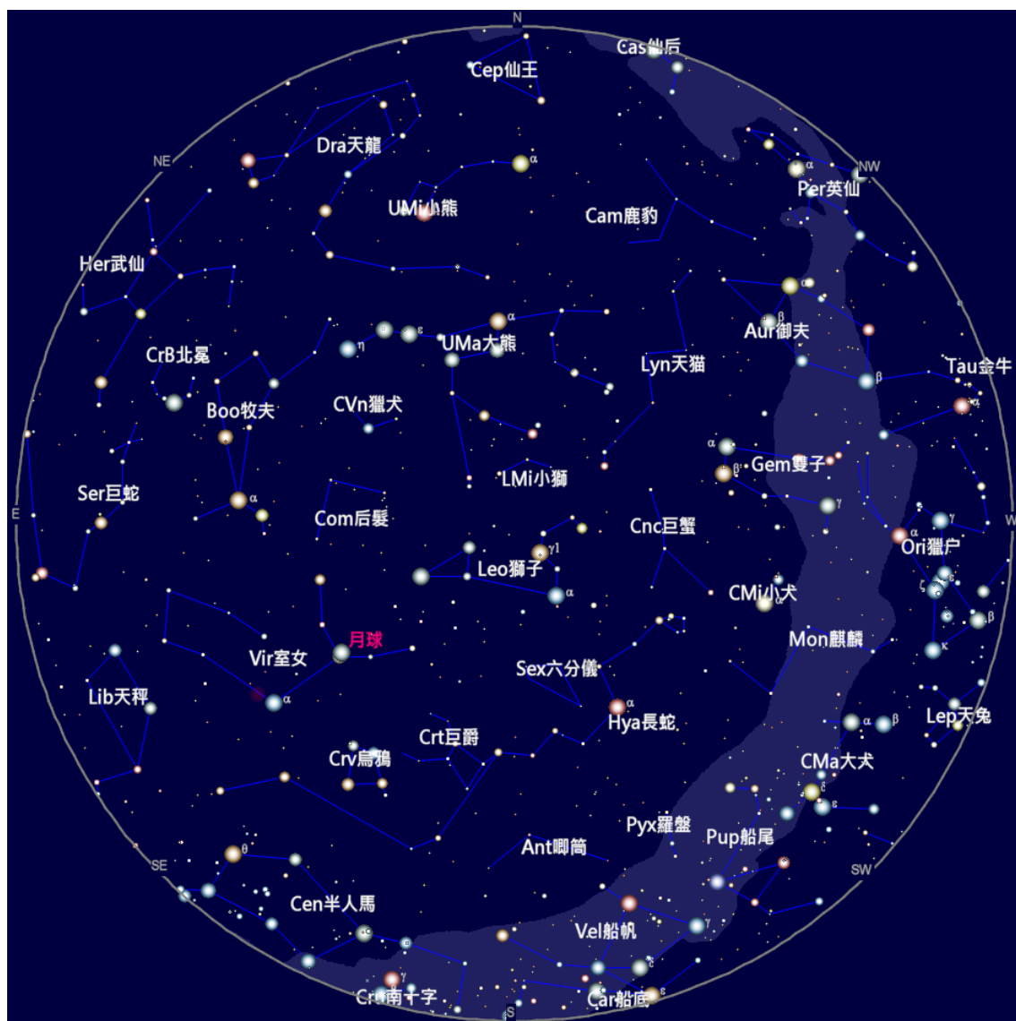
2022 年 4 月 15 日 21:00 的天空
