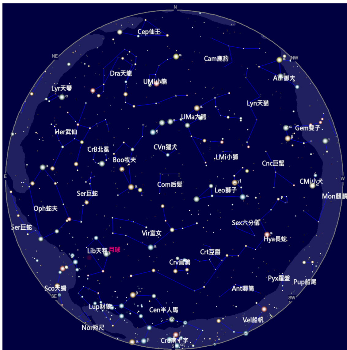
2022 年 5 月 15 日 21:00 的天空
