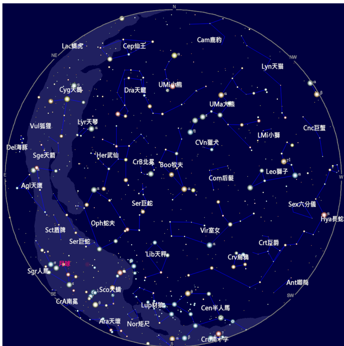
2022 年 6 月 15 日 21:00 的天空
