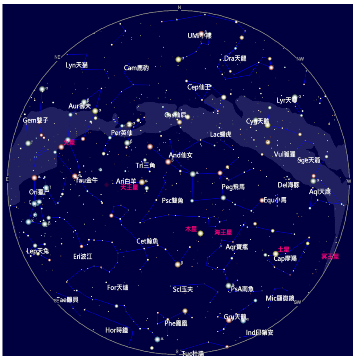
2022 年 11 月 15 日 21:00 的天空
