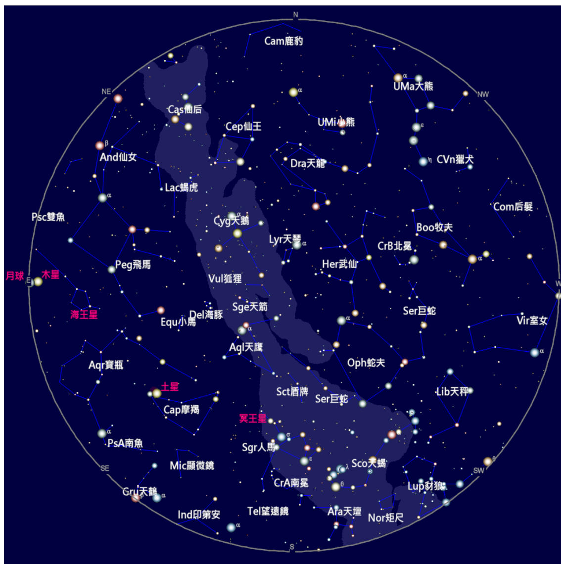
2022 年 8 月 15 日 21:00 的天空
