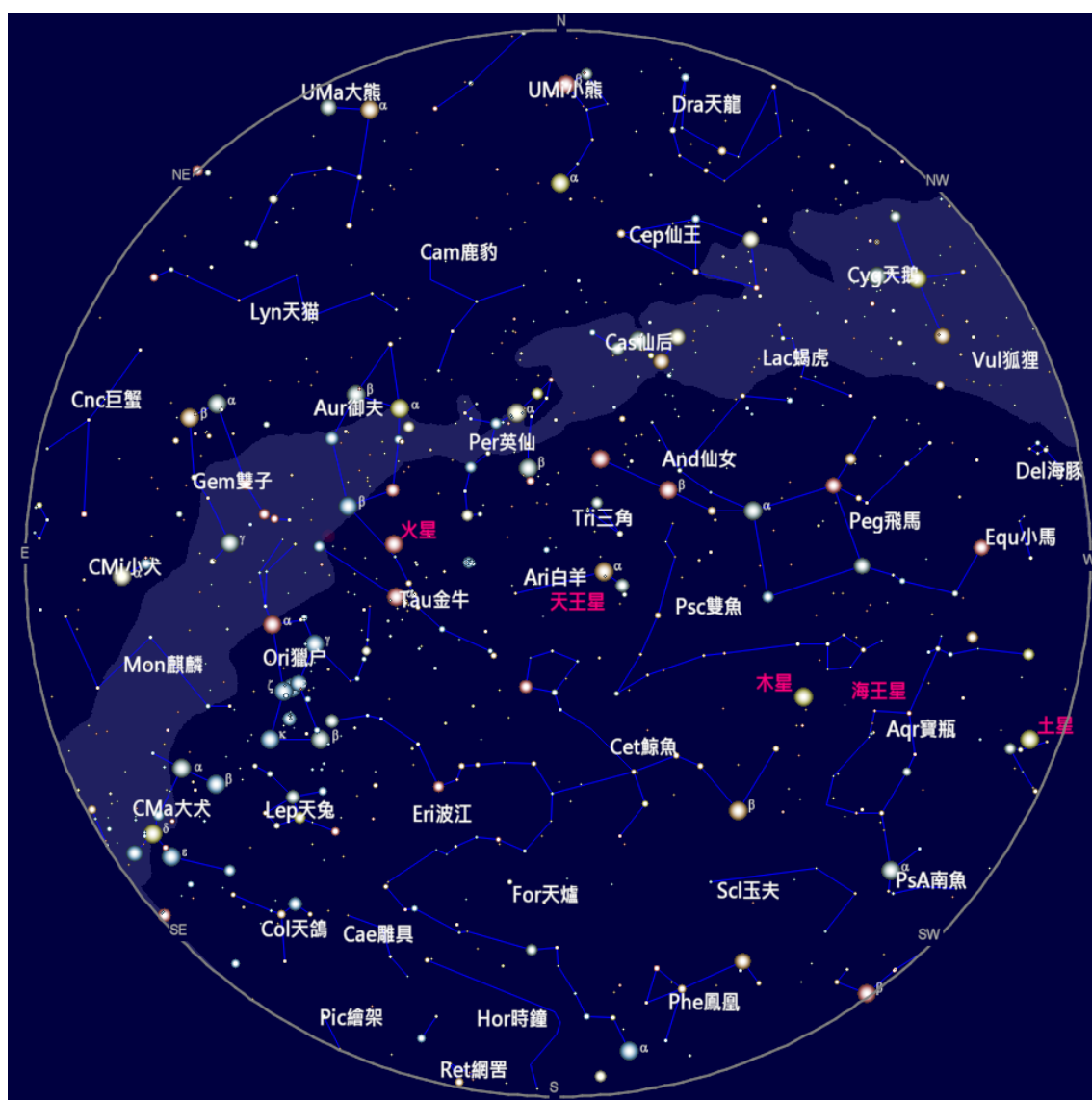
2022 年 12 月 15 日 21:00 的天空
