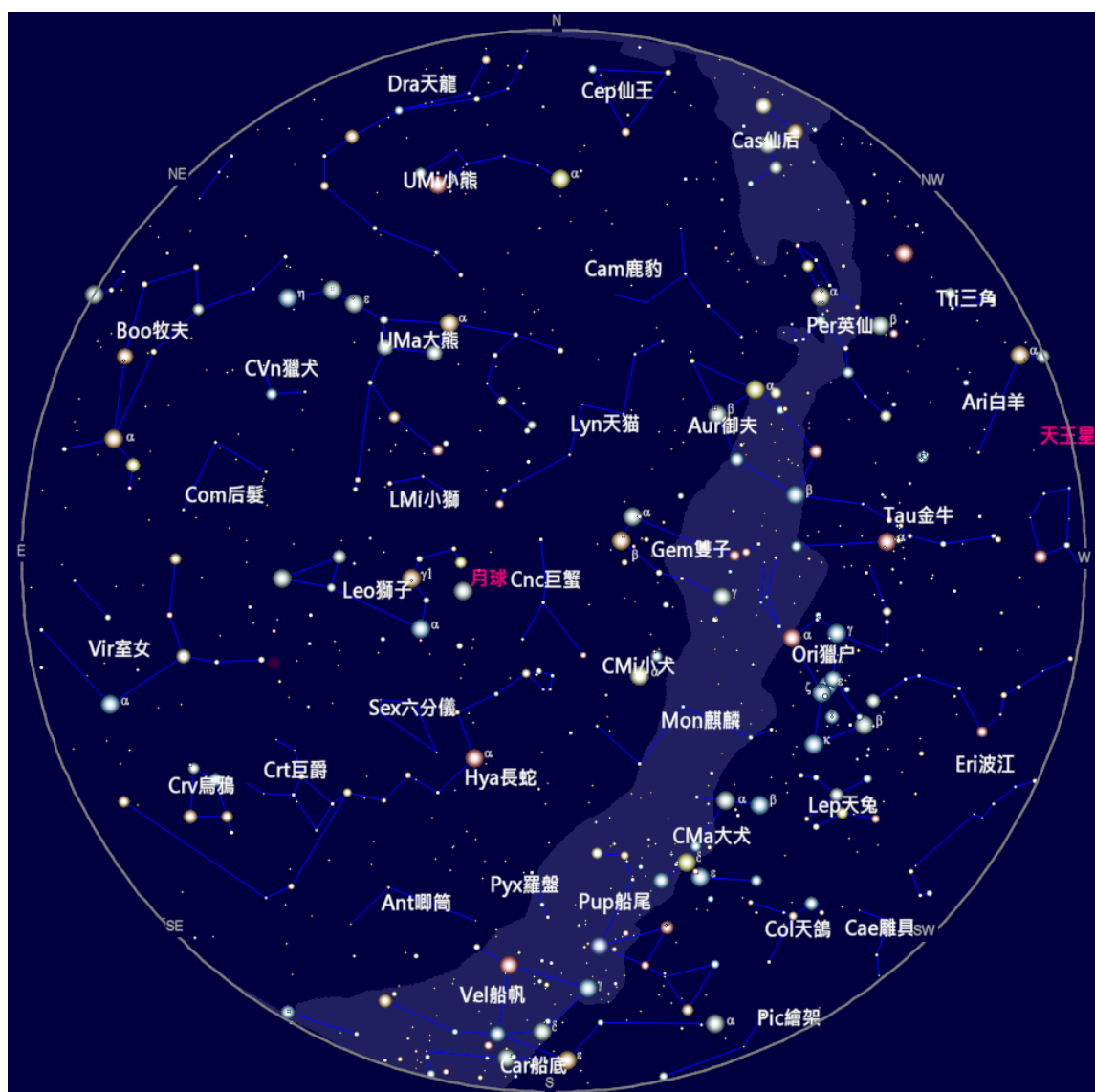
2022 年 3 月 15 日 21:00 的天空
