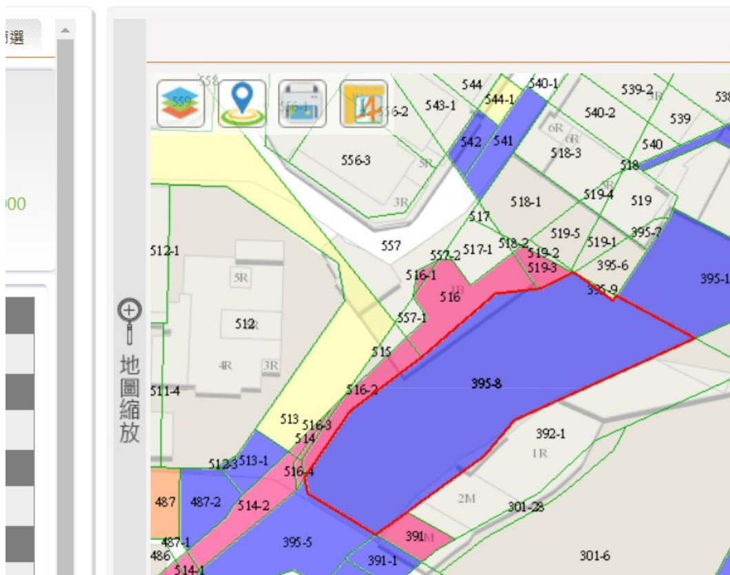
圖別：地籍地形套繪圖(臺北市大同區大龍段一小段 395-8 地號)
