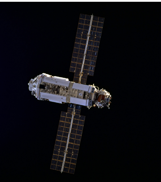
圖3a. 1998年從奮進號太空梭上拍攝的曙光號功能貨艙（Zarya），這也是第一個升空的國際太空站組件。圖片來源：wiki
