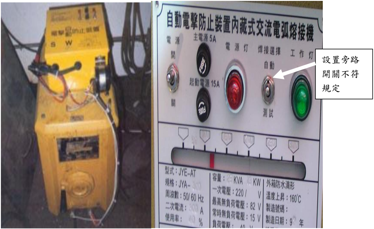
外掛式自動電擊防止裝置 內藏式自動電擊防止裝置
