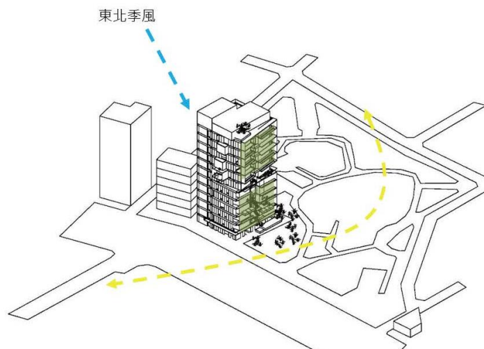
物理環境/服務核阻擋東北風，南向深遮陽及垂直綠化引入西南風
