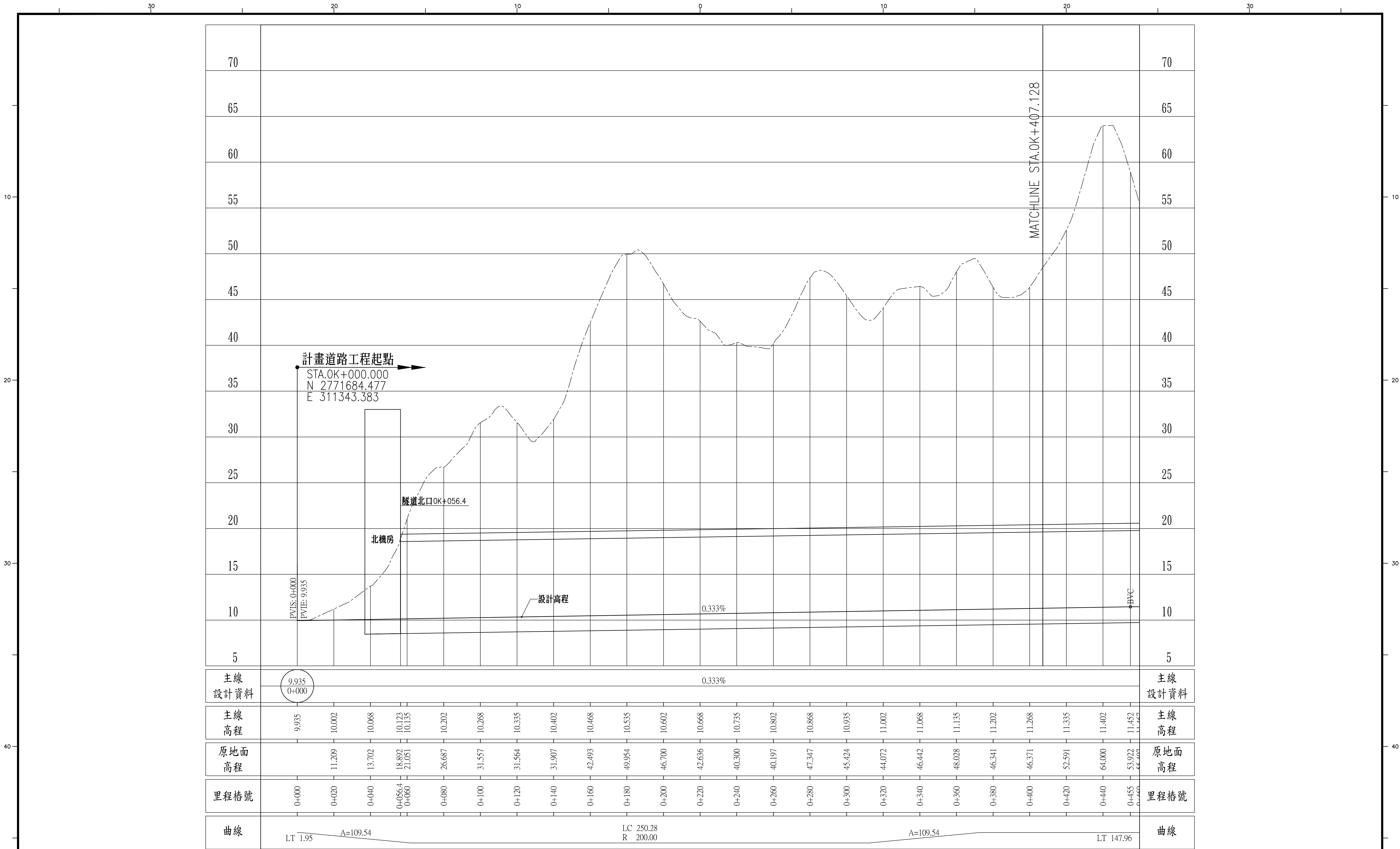
縱面圖(V=1:200、H=1:1000)
