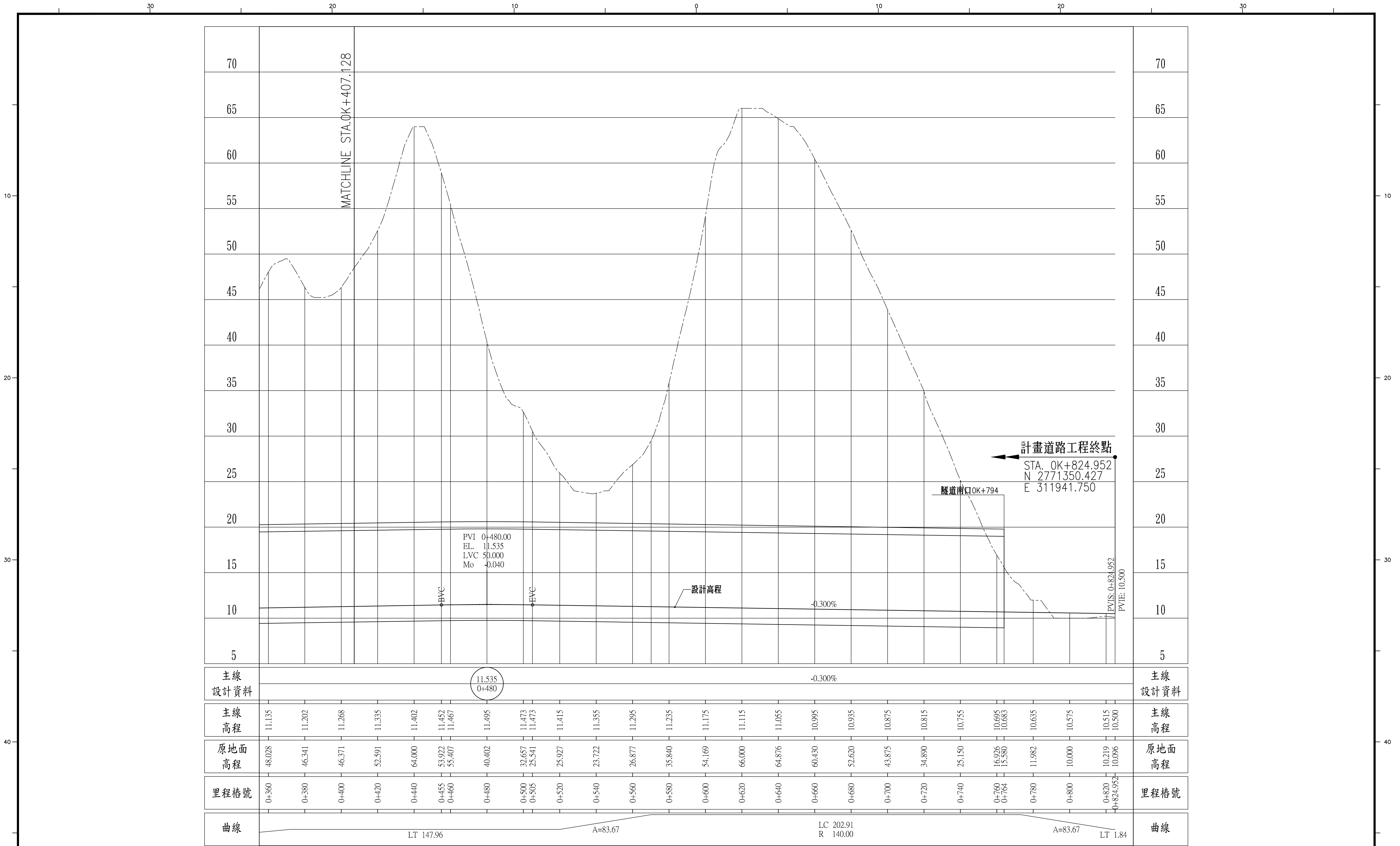
縱面圖(V=1:200、H=1:1000)
