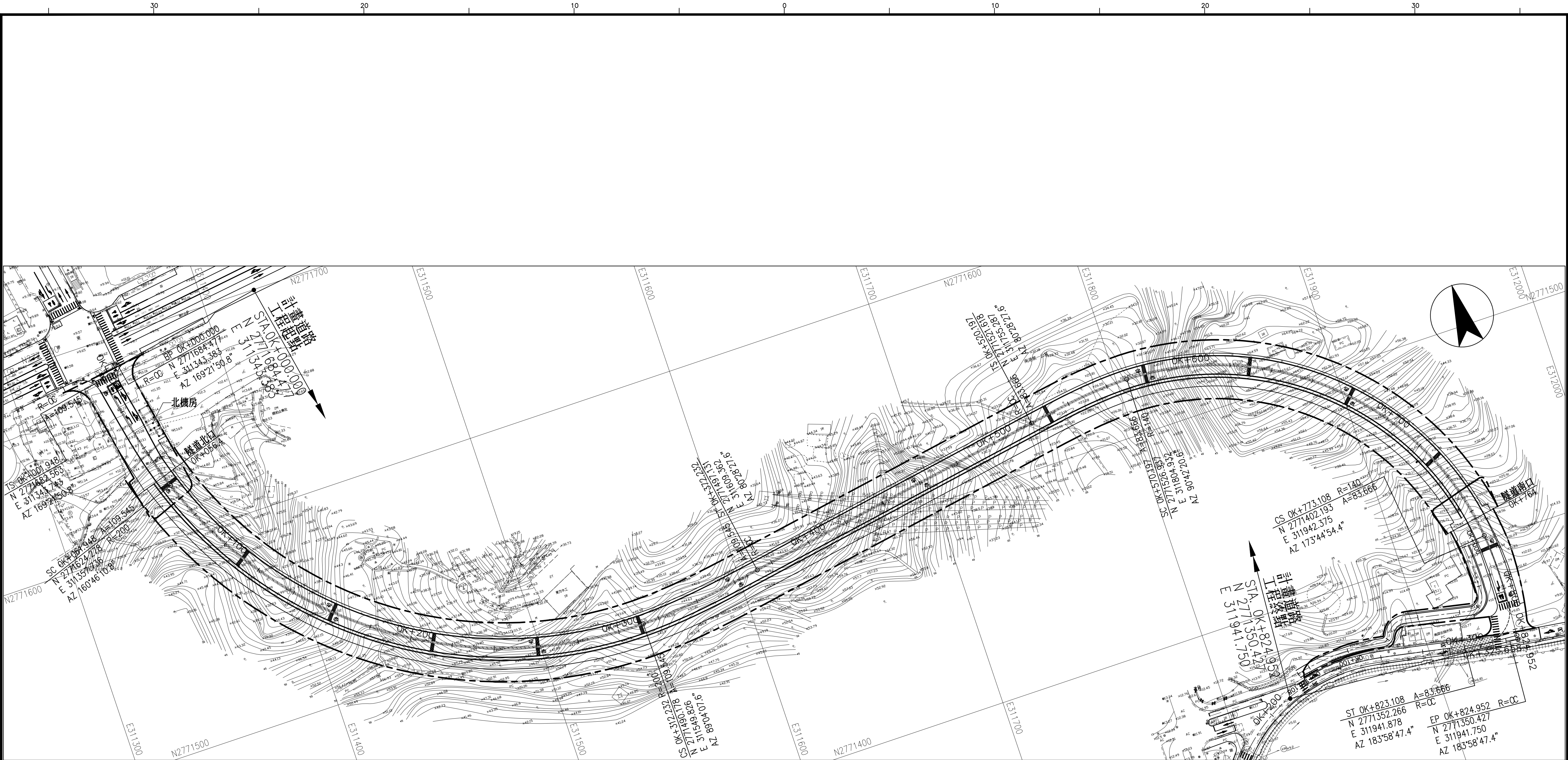
平面圖(S=1:1000)
